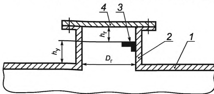
1 — верхняя образующая ТМ; 2 — горловина ТМ; 3 — указатель уровня налива; 4 — крышка горловины
