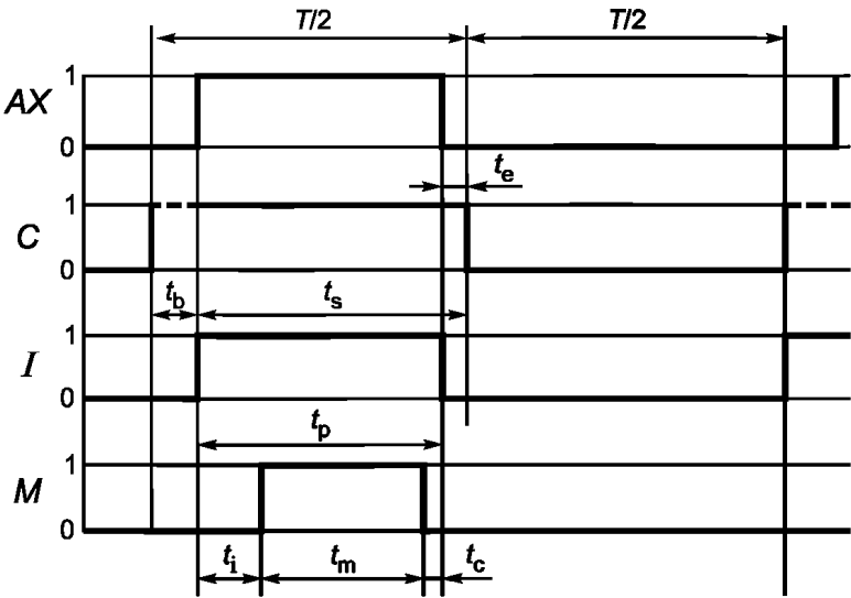
С — испытуемый контакт; I — испытательный ток; M — измерение падения напряжения или контроль нагрузки; T — период испытательного цикла; АХ — вспомогательный контакт; t_b — время, необходимое для достижения устойчивого состояния («дребезг» закончен), составляет не менее 10 мс; t_c — конечное время без наблюдения до отключения тока (например, t_c = 10\% t_p ); t_e — интервал времени между размыканием АХ и С; t_i — начальное время без наблюдения после подачи тока, t_i \leq 40\% t_p и не менее 10 мс; t_m — время измерения падения напряжения в контакте ( U_k ) или контроль нагрузки; t_p — время прохождения тока; t_s — время устойчивого состояния испытуемого контакта
