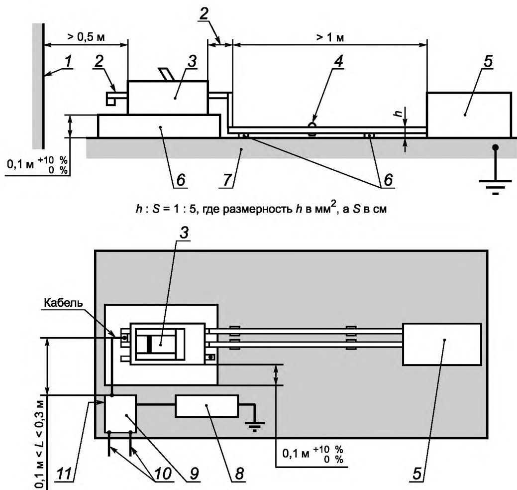
1 — любая другая металлическая часть; 2 — расстояние должно быть минимальным; 3 — испытуемый аппарат; 4 — поперечное сечение S; 5 — трансформатор; 6 — изолирующее основание; 7 — заземляющая пластина; 8 — генератор РЧ; 9 — сеть; 10 — сетевые выводы отключены; 11 — устройство связи/развязки M1; L — общая длина кабеля
