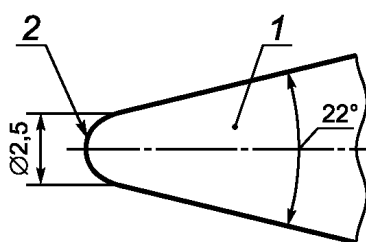
Рисунок 108 — Ударный элемент для проведения испытания по проверке устойчивости к механическим ударам, наносимым предметами с острыми кромками
