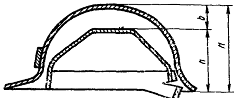
H — высота корпуса каски; h — глубина внутренней оснастки; b — вертикальный безопасный зазор.
