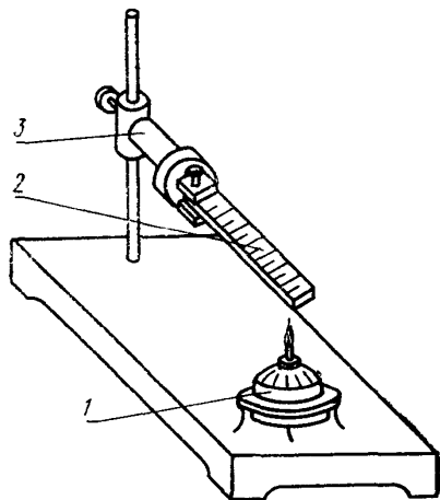
1—спиртовая горелка; 2—испытуемый образец; 3—штатив Черт. 4
