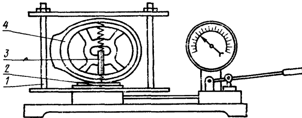
1—приставка; 2—поршень гидравлического пресса; 3—регистратор прогиба; 4—испытываемая каска.
