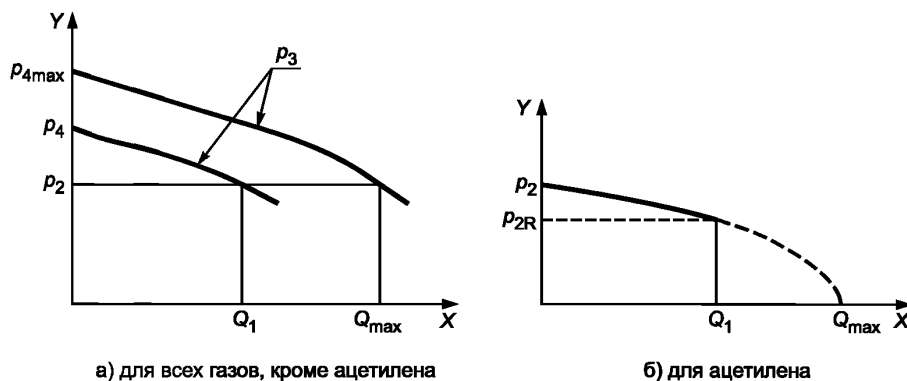
Рисунок 2 — Характеристики расхода
