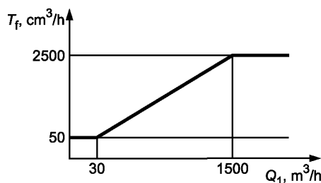
Рисунок 1 — Уровни допустимой внутренней утечки
