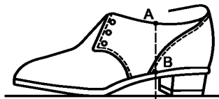
Рисунок 7 — Измерение перекаса берцев
