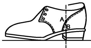
Рисунок 8 — Измерение перекаса накладных задников (задников)
