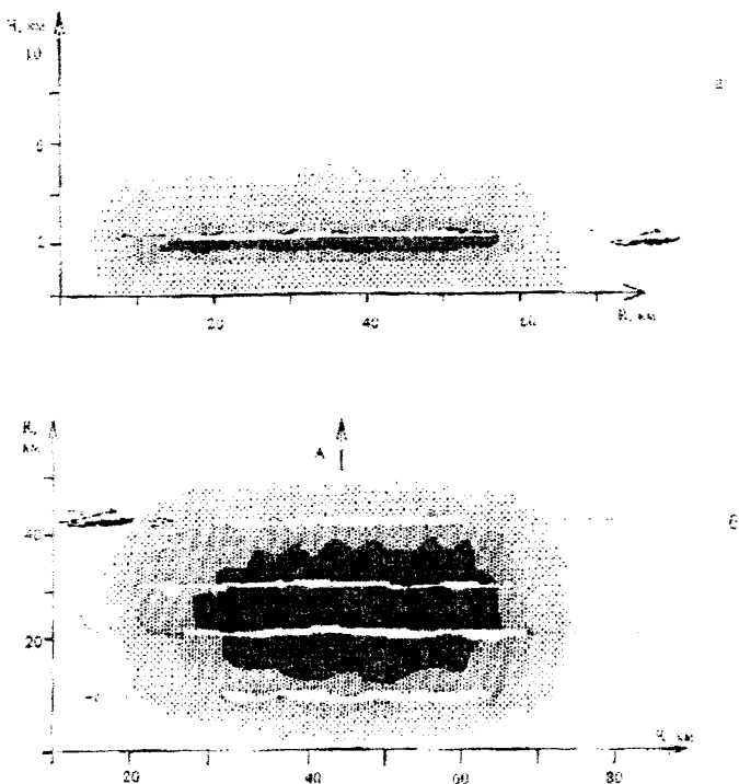
Рис. 8.8 – Схема засева слоисто-дождевой облачности (As-Ns)
