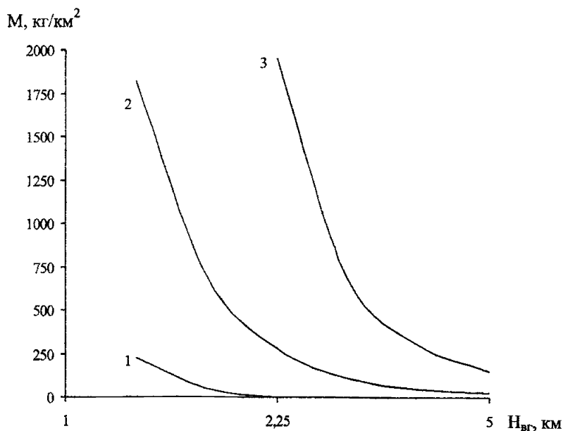
Рис. 8.2 – Зависимость оптимального количества реагента M от H_{\text{вг}} и r_0 . 1 – r_0 = 30 \text{ мкм} , 2 – r_0 = 60 \text{ мкм} , 3 – r_0 = 100 \text{ мкм}
