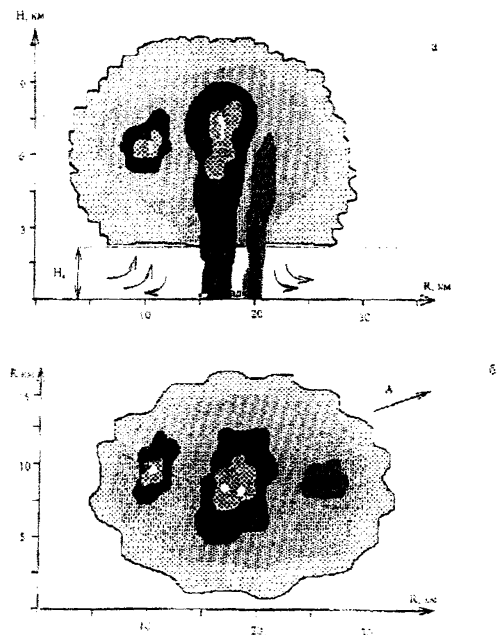
Рис. 8.15 – Схема засева многоячейковой мощной кучево-дождевой облачности (Сб) а – вертикальный разрез облака, б – горизонтальный разрез облака
