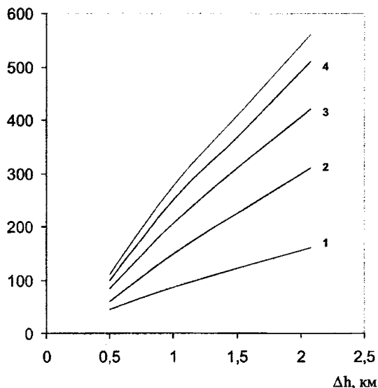
Рис. 8.4 – Номограммы для расчета величины R_2 (а) по известным \bar{q} и \Delta h^* = h_0 - H_{н.г.} : 1, 2, 3, 4 – \bar{q} = 0,4; 0,3; 0,2; 0,1 \text{ г/м}^3 соответственно и величины R_3 (б) по известным величинам H_{н.г.} и осредненных величин относительной влажности ( \bar{f} ) между землей и H_{н.г.} : 1, 2, 3, 4, 5 – \bar{f} = 90; 80; 70; 60; 50 \% соответственно.
