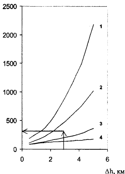
Рис. 8.4 – Номограммы для расчета величины R_2 (а) по известным \bar{q} и \Delta h^* = h_0 - H_{н.г.} : 1, 2, 3, 4 – \bar{q} = 0,4; 0,3; 0,2; 0,1 \text{ г/м}^3 соответственно и величины R_3 (б) по известным величинам H_{н.г.} и осредненных величин относительной влажности ( \bar{f} ) между землей и H_{н.г.} : 1, 2, 3, 4, 5 – \bar{f} = 90; 80; 70; 60; 50 \% соответственно.
