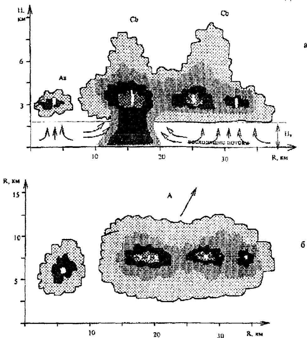
Рис. 8.16 – Схема засева слоисто-кучево-дождевой облачности системы Ns-As-Cb а – вертикальный разрез облака, б – горизонтальный разрез облака
