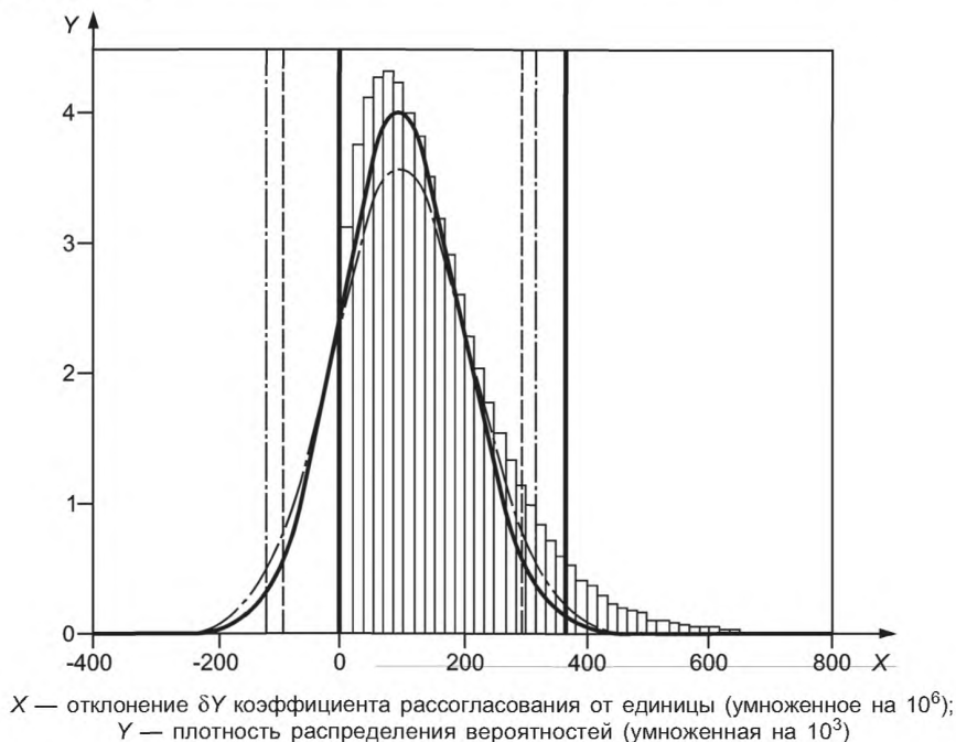
Рисунок 13 — То же, что и на рисунке 11, но для x_1 = 0,010 и с двумя кривыми, полученными способом оценивания по GUM (высокий пик — учтены только члены 1-го порядка; низкий пик — учтены члены более высокого порядка)
