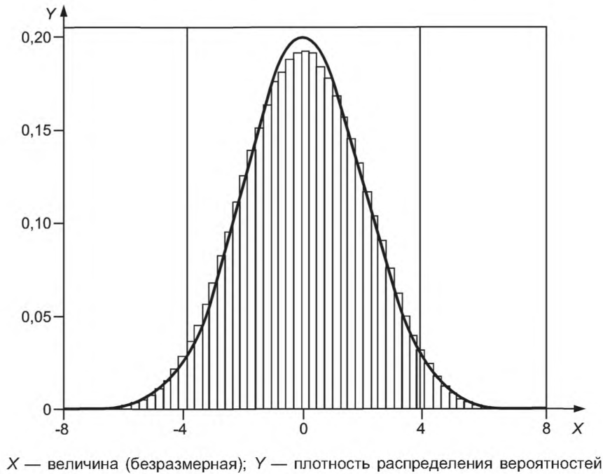
Рисунок 8 — То же, что и на рисунке 6, но для равномерно распределенных входных величин с одинаковыми математическими ожиданиями и одинаковыми стандартными неопределенностями
