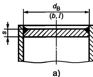
а) односторонняя сварка
