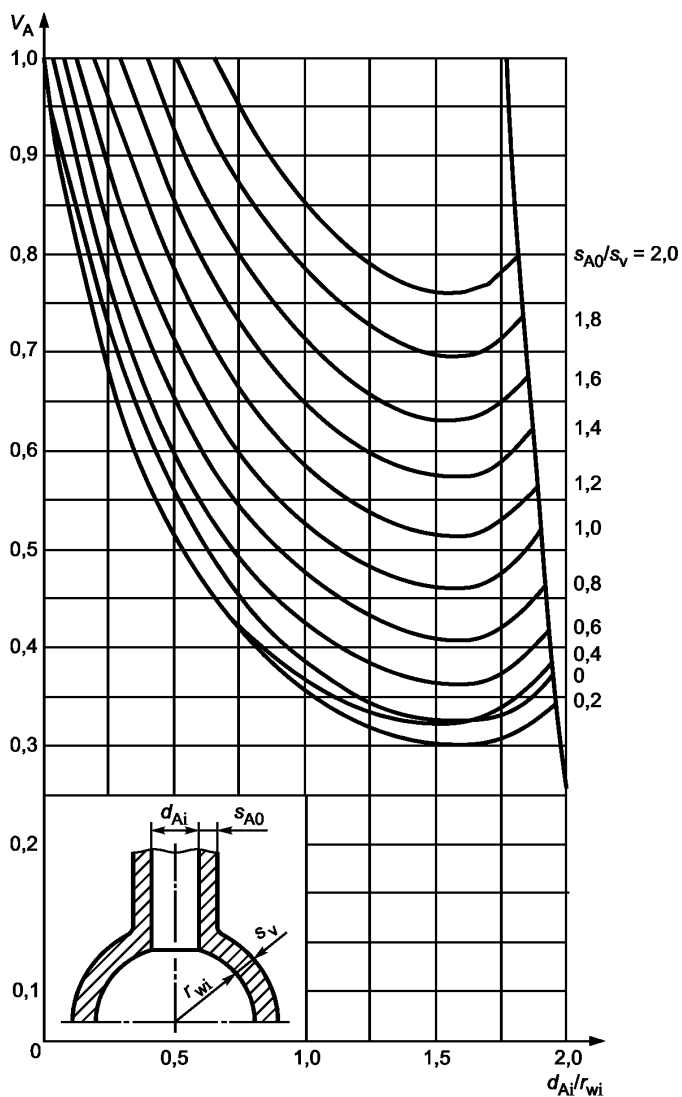
Рисунок В.13 — Значения коэффициента эффективности для сферических оболочек с вертикальным патрубком в зависимости от d_{Ai}/r_{wi} и s_{A0}/s_v при постоянном значении s_v/r_{wi}
