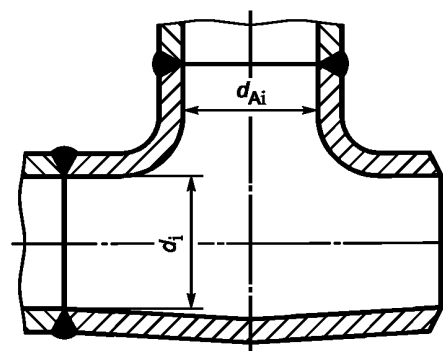
Рисунок А.5 — Патрубок, выполненный объемной штамповкой
