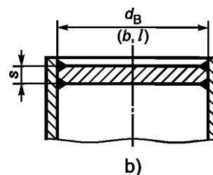
б) двусторонняя сварка
