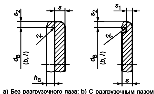
Рисунок D.1 — Сварные днища
