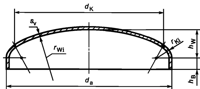
Рисунок В.1 — Выпуклое днище
