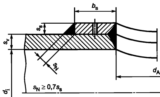
Рисунок А.7 — Отверстие с упрочняющим слоем (при температуре \leq 250\text{ }^{\circ}\text{C} )
