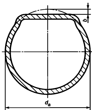
Рисунок Е.2 — Уплощение цилиндрических оболочек
