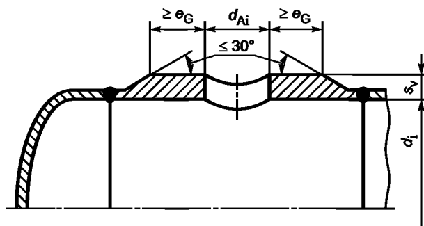
Рисунок А.1 — Усиление посредством увеличения толщины стенки основной оболочки с отверстием
