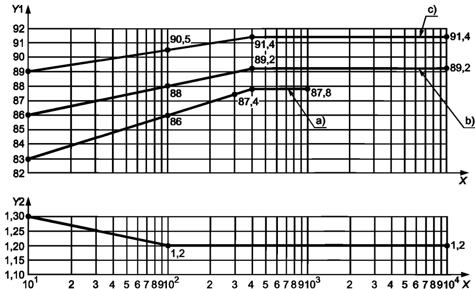
Y1 — КПД; Y2 — коэффициент избытка воздуха; X — тепловая мощность P_n , кВт a) \eta_{K^*} отопительный котел, 30 % P_n ; b) \eta_{K^*} отопительный котел, P_n ; c) \eta_{K^*} низкотемпературный отопительный котел, P_n и 30 % P_n (только для котлов мощностью до 1000 кВт)
