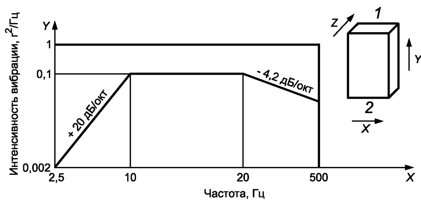
Рисунок D.2 — Испытания на транспортирование
