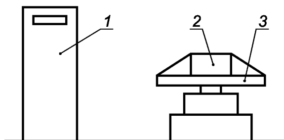
Рисунок D.1 — Испытания на виброустойчивость
