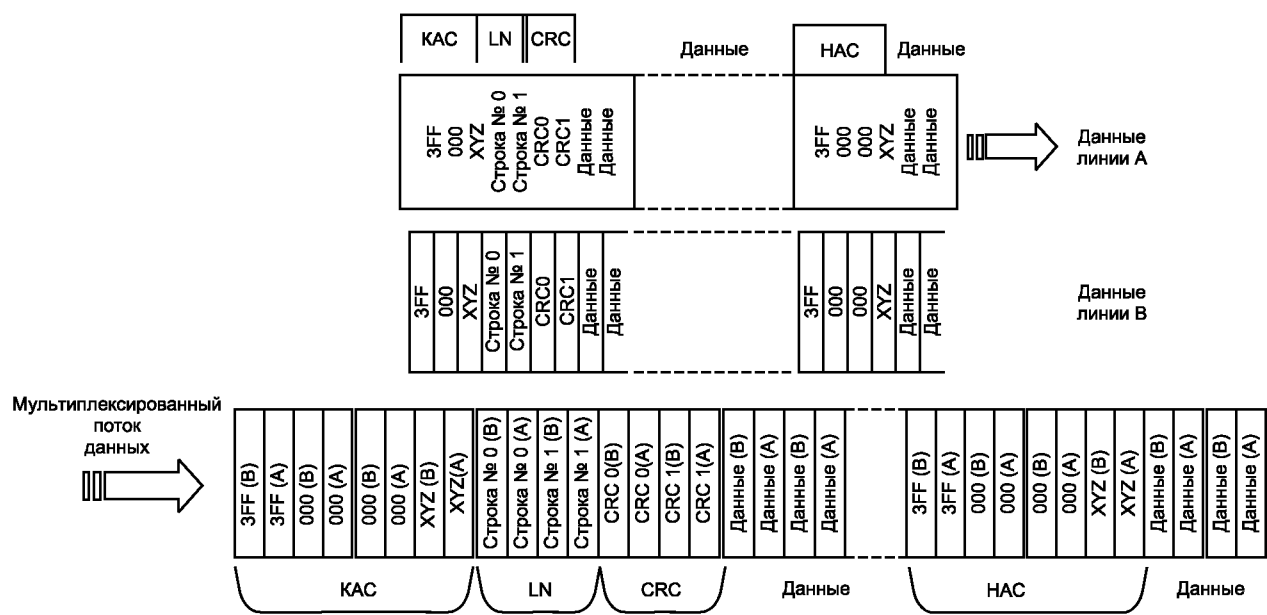
Рисунок 13 — Мультимплексирование двух линий в одну
