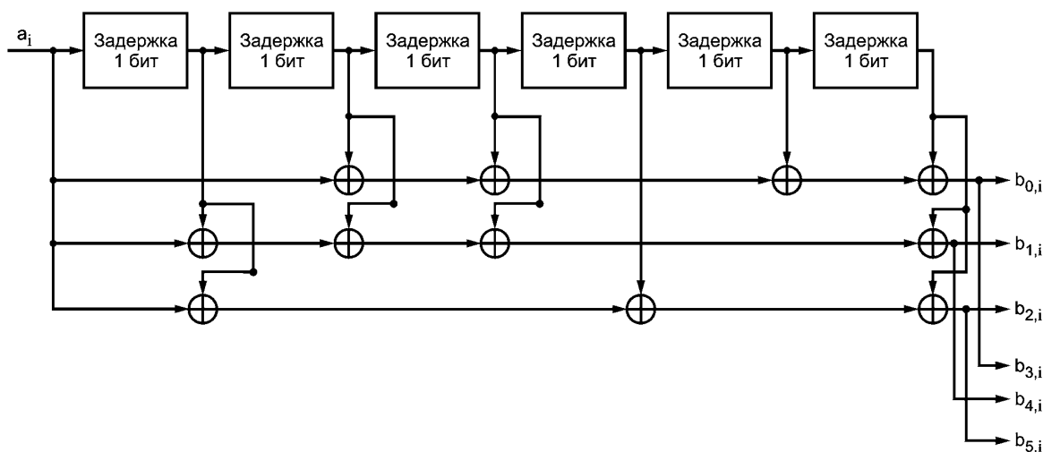
Рисунок 34 — Сверточный кодер
