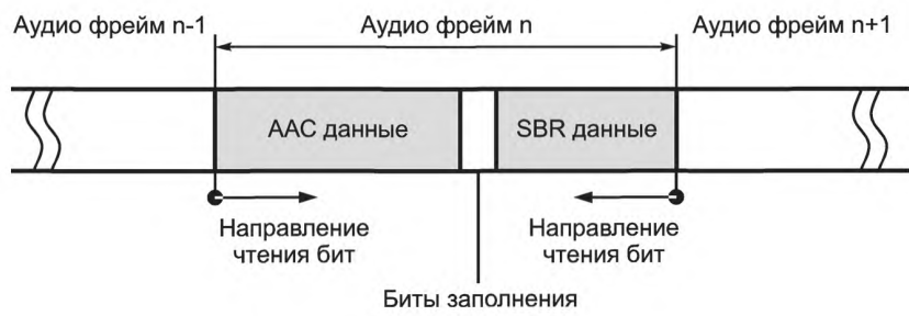
Рисунок 5 — Фрейм AAC + SBR
