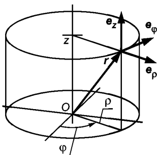
Рисунок 2 — Цилиндрическая система координат (правосторонняя)
