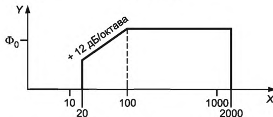
Рисунок 3 — Форма спектральной мощности ускорения для электродинамического вибростенда (по ИСО 5344)
