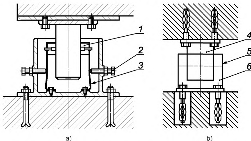
1 — фрикционная обшивка; 2 — регулировочный винт; 3 — пружина сжатия; 4 — поршень; 5 — корпус; 6 — жидкость
