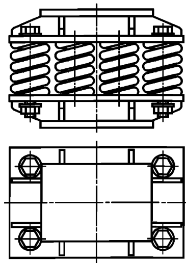
Рисунок А.3 — Типичная подвеска из цилиндрических винтовых пружин сжатия
