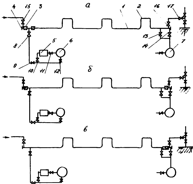
Рис.5. Схема испытания трубопровода жидкостью с пониженной температурой замерзания:
