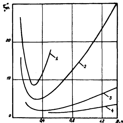
Рис.2. Зависимость времени прокачки воды с температурой T_{\text{в}} = 50^{\circ}\text{C} для эталонного трубопровода от его диаметра при суммарной производительности Q наполнительных агрегатов, \text{м}^3/\text{ч} :
