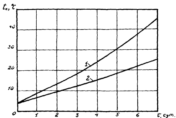
Рис.1. Зависимость начальной температуры воды от продолжительности испытания при температуре наружного воздуха:
