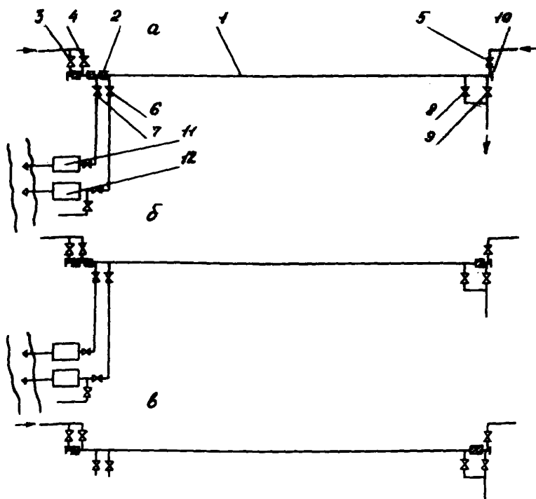
Рис.3. Схема испытания подземных трубопроводов без теплоизоляции:
