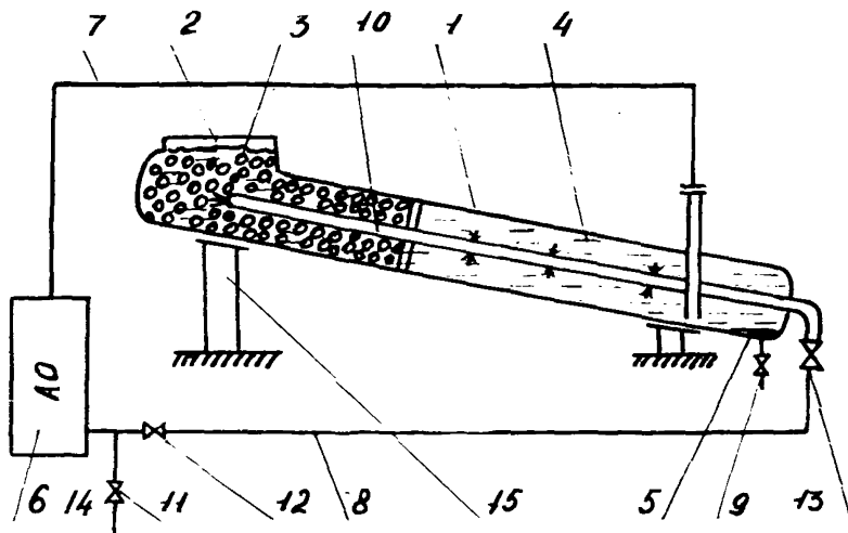
Рис.4. Схема установки приготовления раствора хлористого кальция:
