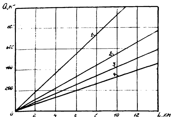
Рис.3. Зависимость объема прокачиваемой воды Q от длины участка L при температуре наружного воздуха t_g = -40^{\circ}\text{C} и начальной температуре воды t_n :
