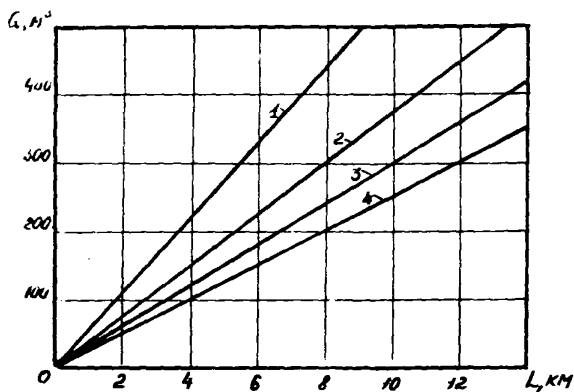
Рис.2. Зависимость объема прокачиваемой воды Q от длины участка L при температуре наружного воздуха t_g = -20^\circ\text{C} и начальной температуре воды t_n :
