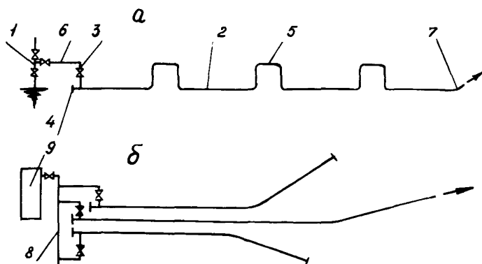
Рис. I. Схема продувки трубопровода:
