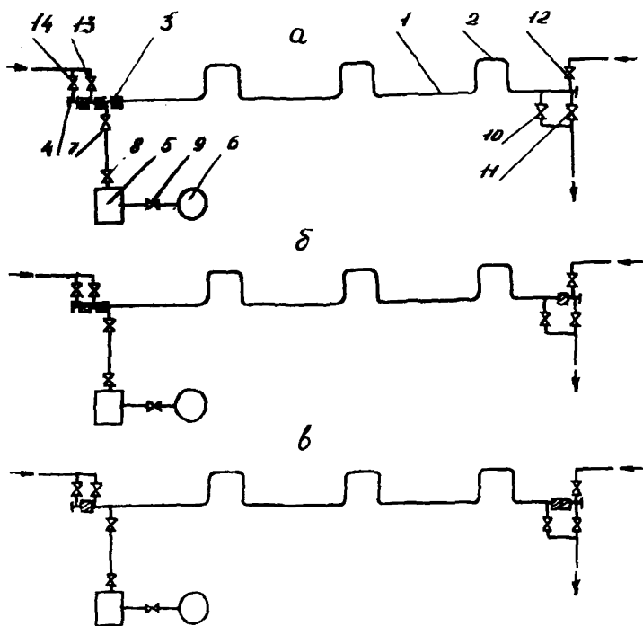
Рис.2. Схема испытания трубопровода подогретой водой: а-заполнение трубопровода с пропуском разделителя; б-подъем давления, испытание; в-удаление воды; 1-трубопровод; 2-компенсатор; 3-разделитель; 4-заглушка; 5-наполнительно-опрессовочная станция; 6-емкость горячей воды; 7,8,9,10,11 - задвижки; 12,13,14 - краны
