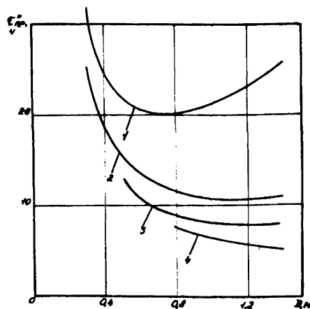
Рис.1. Зависимость времени прокачки воды с температурой T_{\text{в}} = 50^{\circ}\text{C} для эталонного трубопровода от его диаметра при суммарной производительности Q наполнительных агрегатов, \text{м}^3/\text{ч} :
