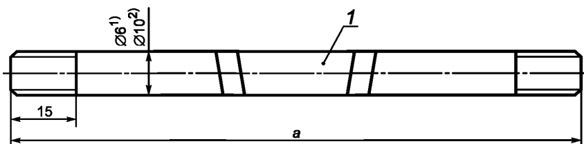
1 — металл сварного шва; а = 130 для кристаллизационного растрескивания, 110 — для ликвационного растрескивания
