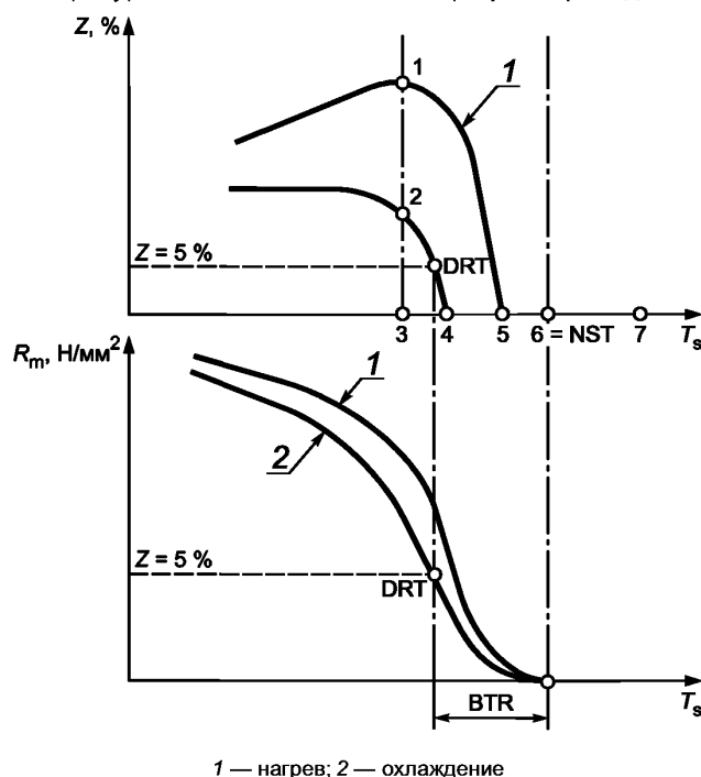
Рисунок 2 — Графики, построенные по результатам испытания
