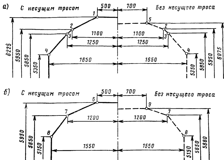
Рис. 2. Минимальное внутреннее очертание В2 верхней части существующих сооружений на электрифицированных линиях:
