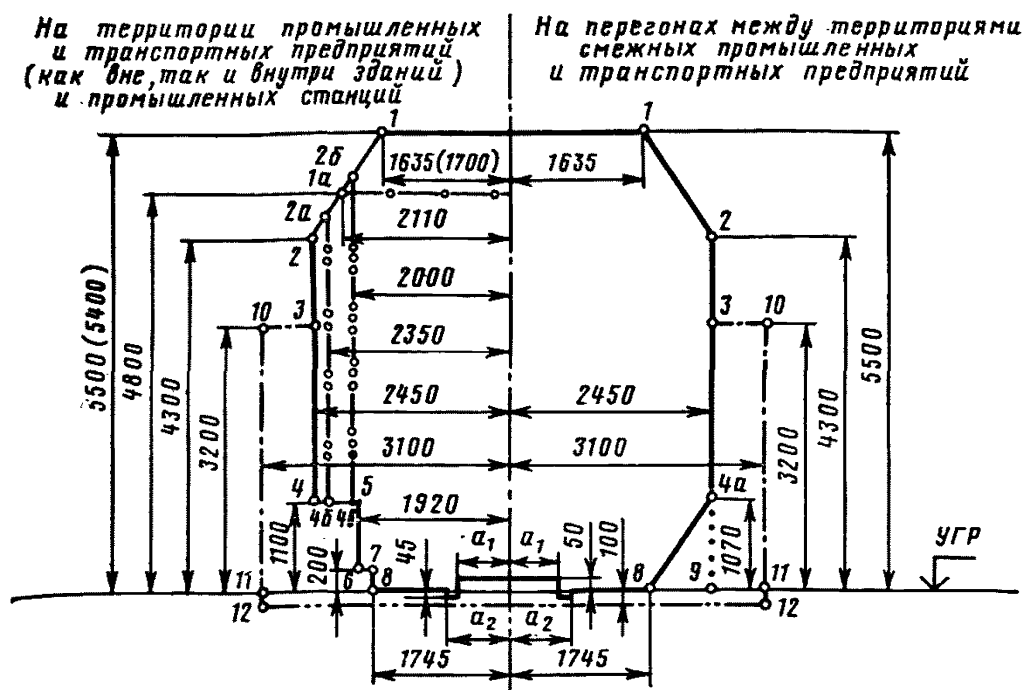
Рис. П.1.2. Габарит приближения строений Сп:
