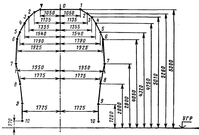
Рис. 8. Контрольное очертание сооружений Цп для пропуска подвижного состава габарита Тц при скорости движения 40 км/ч и менее
