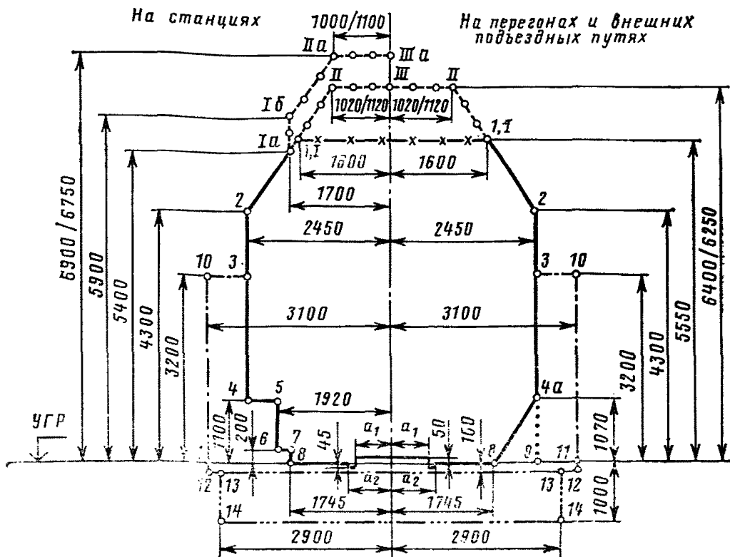
Рис. П.1.1. Габарит приближения строений С:
