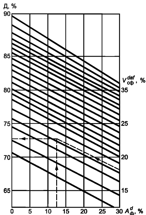
Рисунок 4 — Номограмма для определения добавки инертной пыли ( D )
