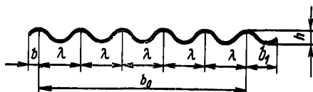
Профиль листа
