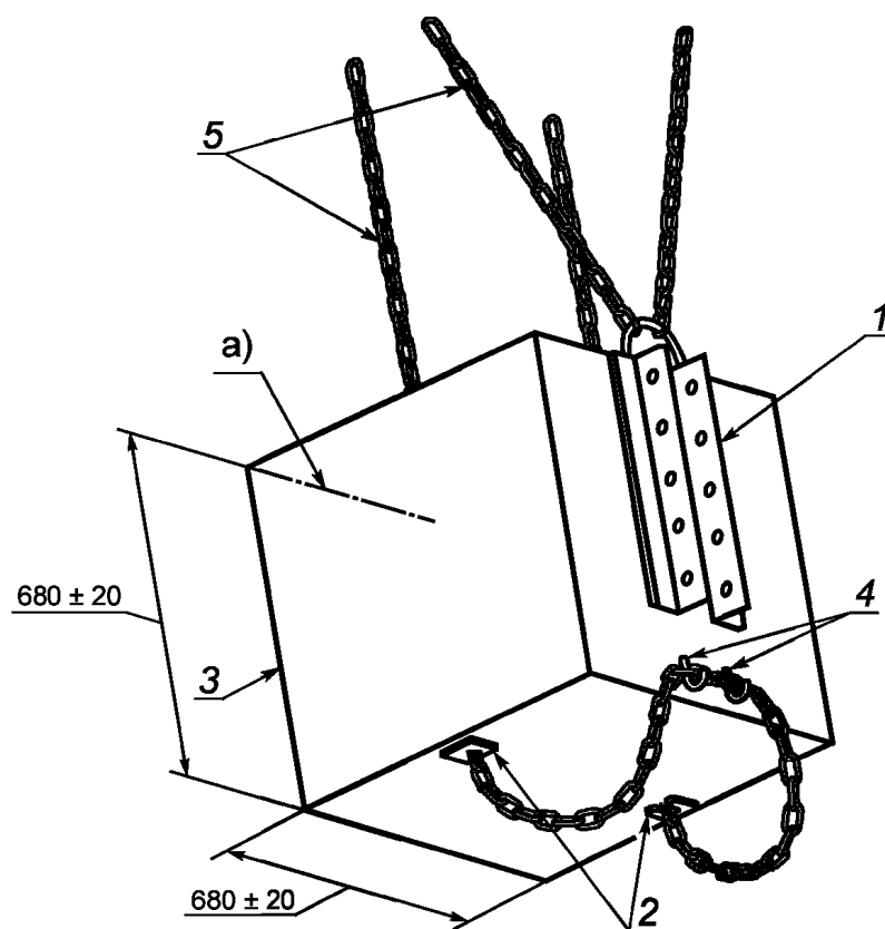
Рисунок 6 — Устройство подвеса блока маятника
