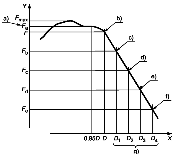
Рисунок 14 — Статическая нагрузка — деформация, при которой испытания с перегрузкой продолжаются
