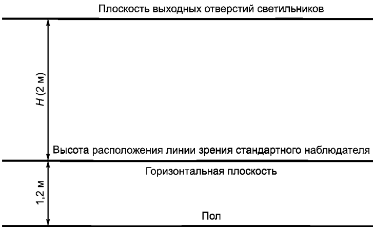
Рисунок 4 — Размеры стандартного модуля в разрезе
