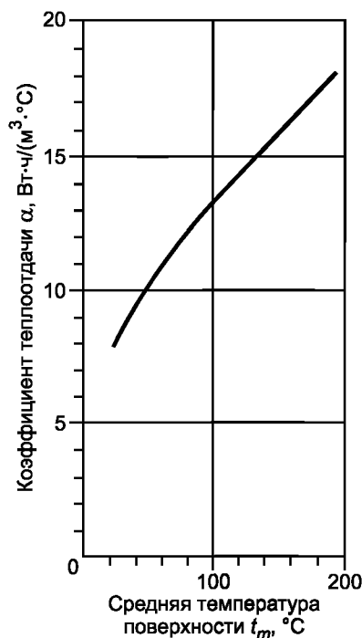
Рисунок А.4 — Значения полной теплоотдачи \alpha радиацией и конвекцией горизонтальным и вертикальным поверхностям при окружающей температуре t_L = 20 °C в зависимости от средней температуры поверхности t_m
