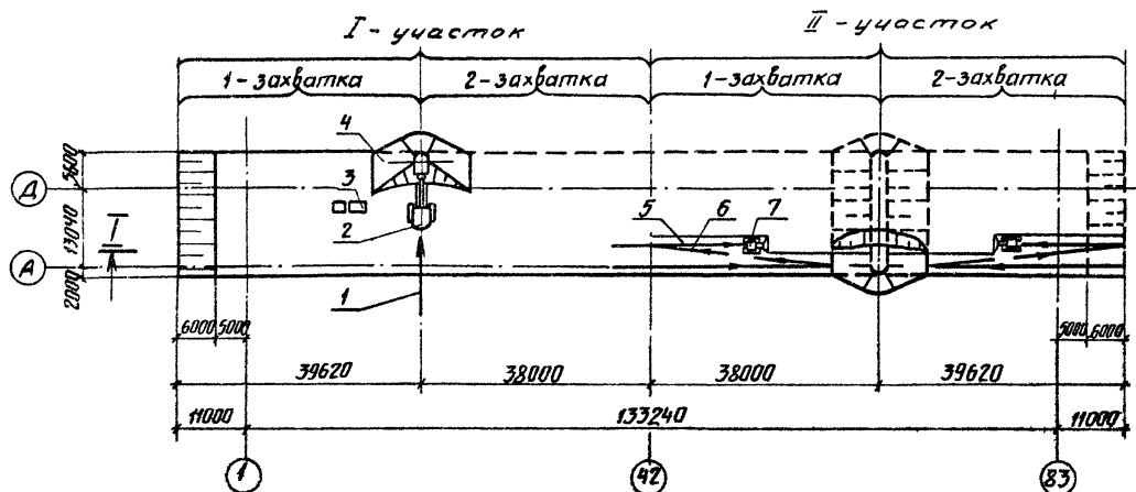
Рис.3. Схема разработки котлована: 1-рабочая проходка; 2-экскаватор Э-652; 3-автосамосвал МАЗ-205; 4-отвал грунта; 5-рабочая проходка бульдозера; 6-холостая проходка бульдозера; 7-бульдозер Д-271
