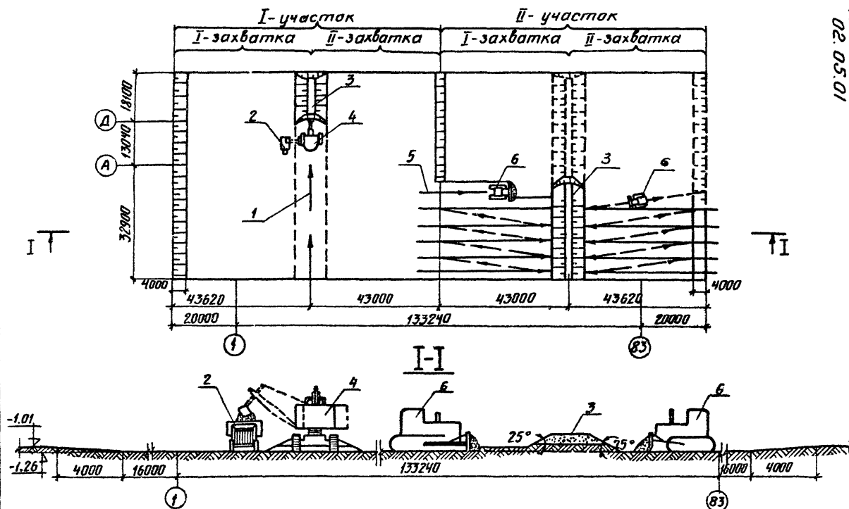
Рис.2. Схема срезки растительного слоя: 1-рабочая проходка экскаватора; 2-автосамосвал МАЗ-205; 3-отвал грунта; 4-экскаватор 3-652; 5-рабочая проходка бульдозера; 6-бульдозер Д-271
