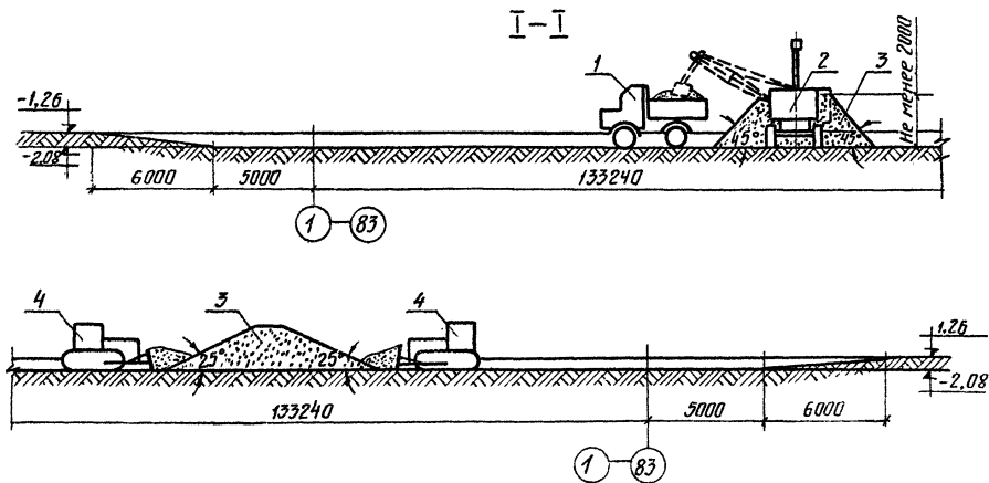
Рис.4. Схема разработки котлована: 1-автосамосвал МАЗ-205; 2-экскаватор Э-652; 3-отвал грунта; 4-бульдозеры Д-271
