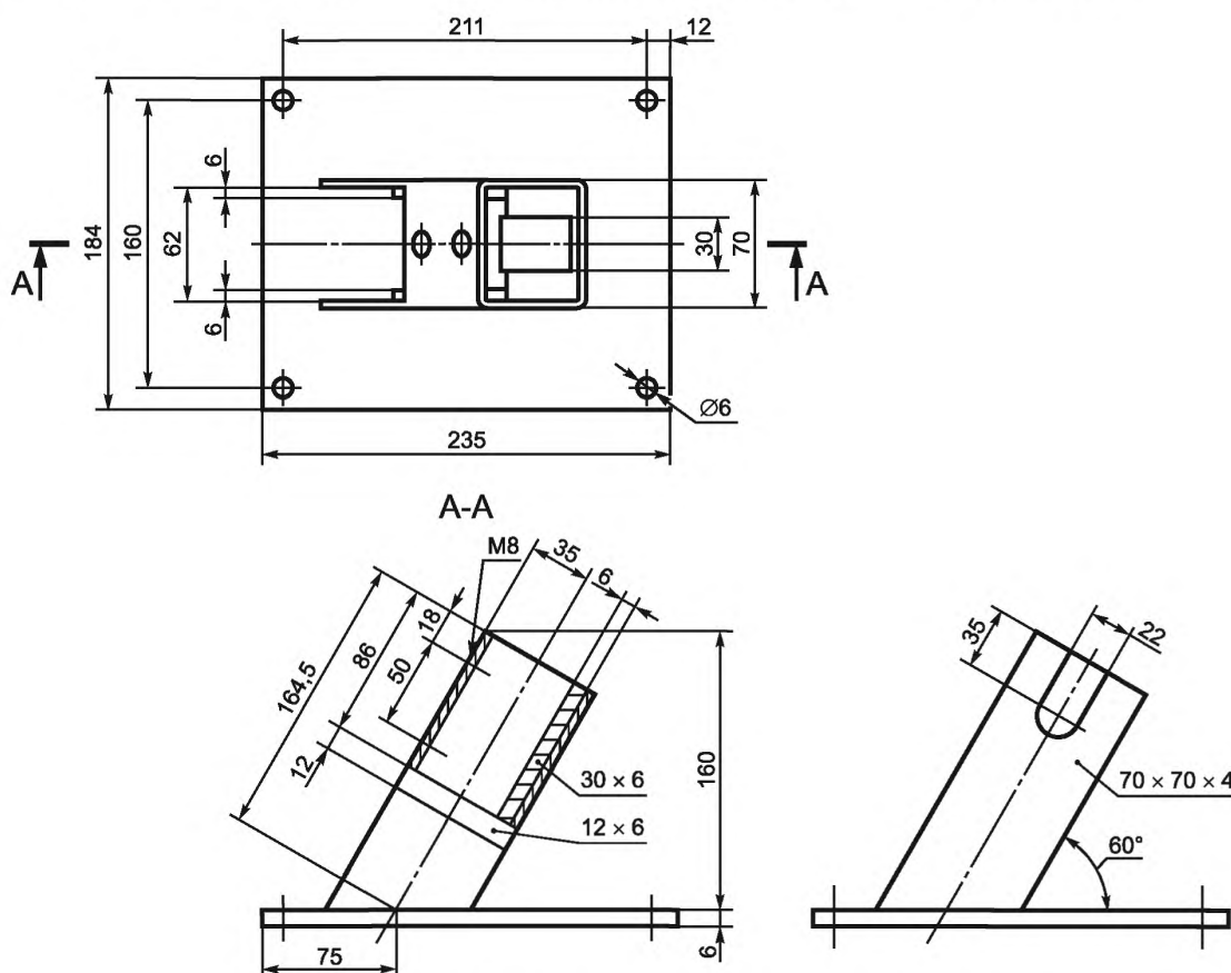
Рисунок 3 — Опорный стенд
