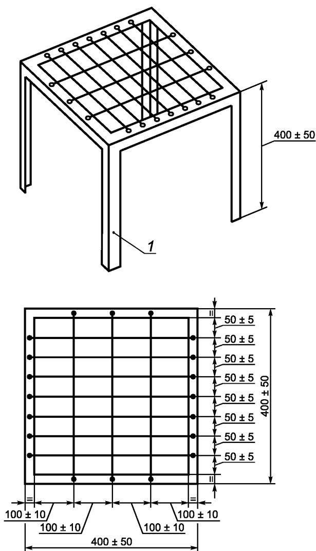
Рисунок 1 — Испытательный стенд
