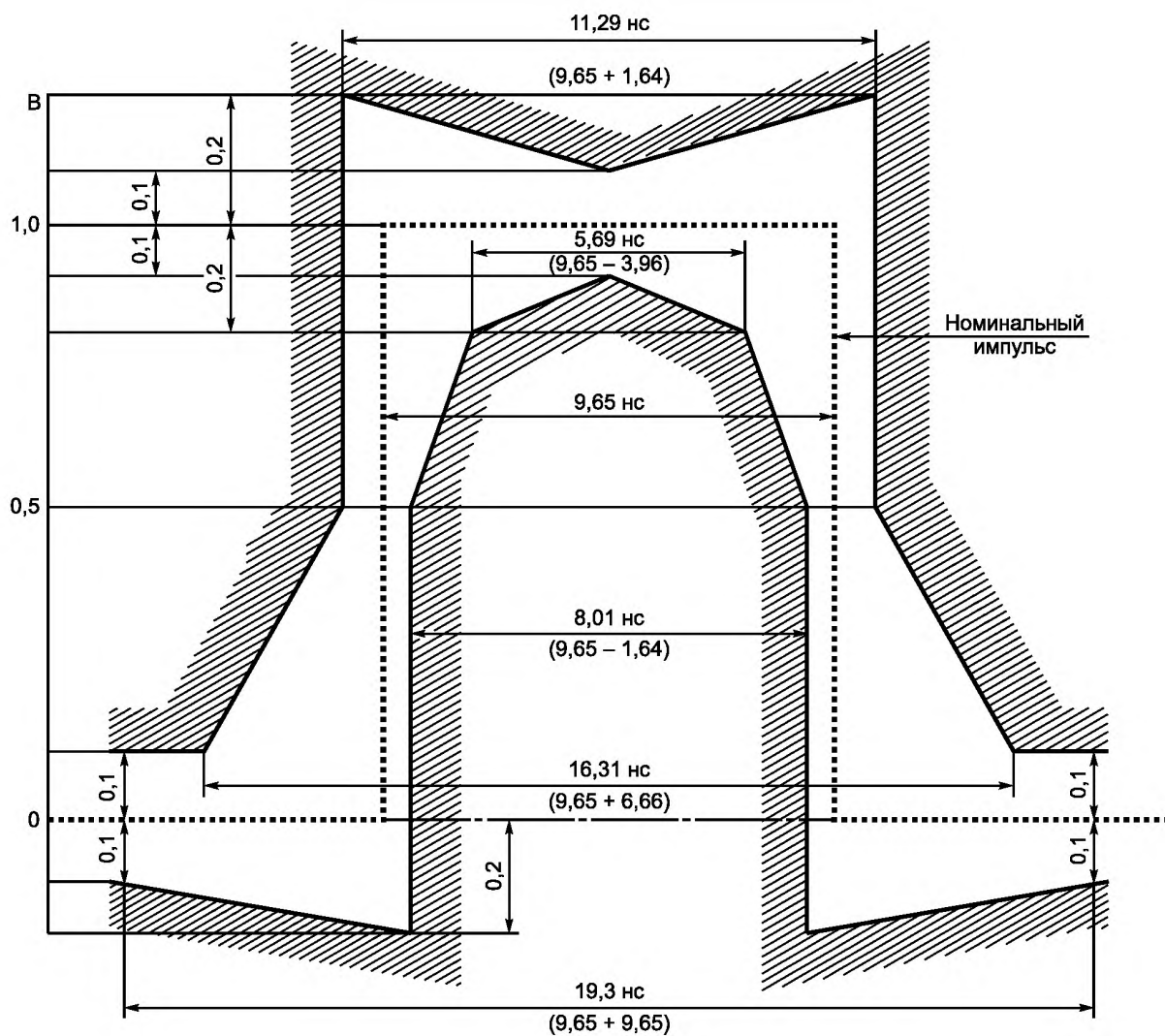
Рисунок Б.1 — Маска импульса 51840 кбит/с (HDB2; HDB3)
