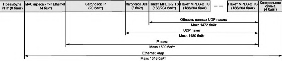
Рисунок 4 — Формат пакетов Ethernet type II
