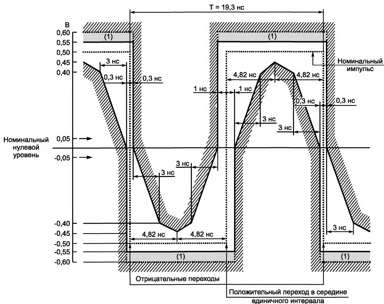
Рисунок Б.3 — Маска импульса 51840 кбит/с 1 (CMI; «0»)
