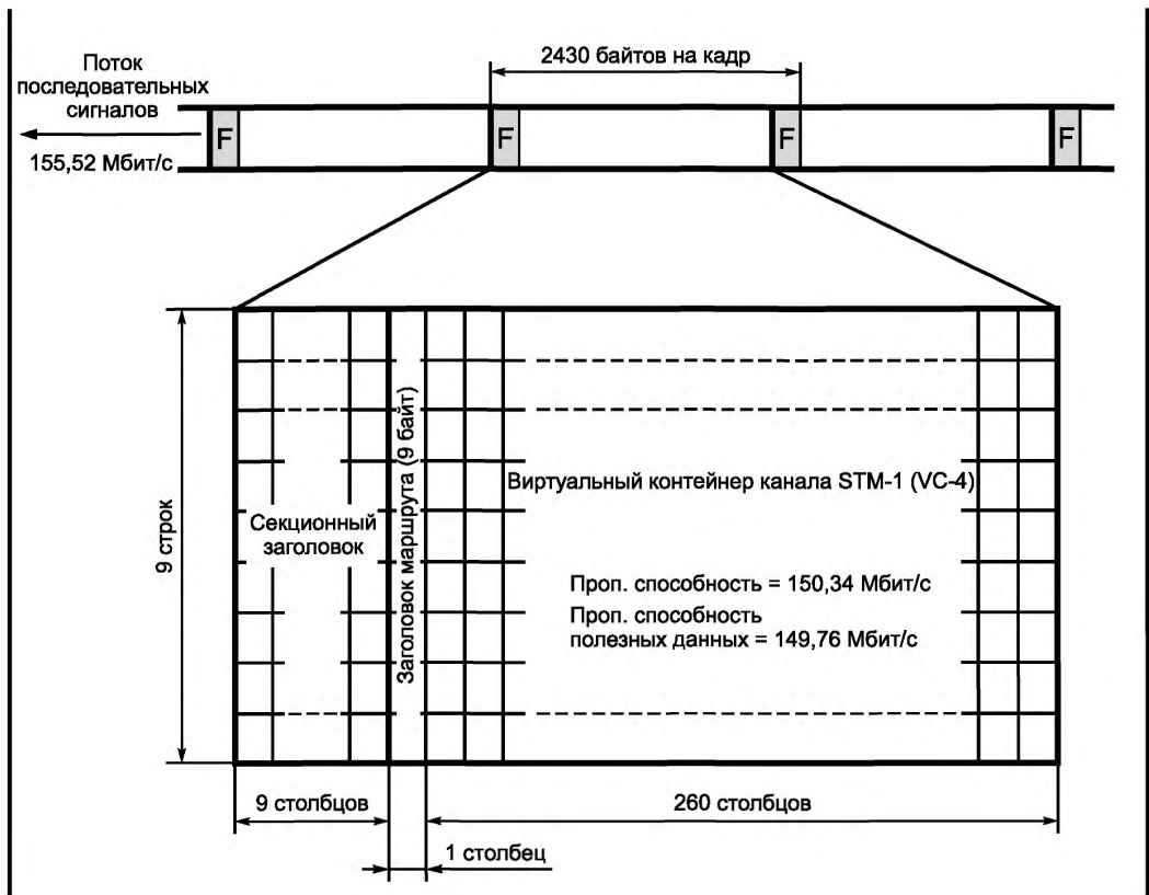
Рисунок 11 — Структура кадров канала STM-1
