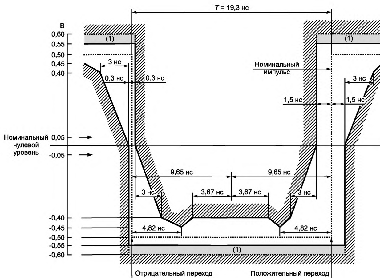
Рисунок Б.2 — Маска импульса 51840 кбит/с 1, 2 (CML; «1»)
