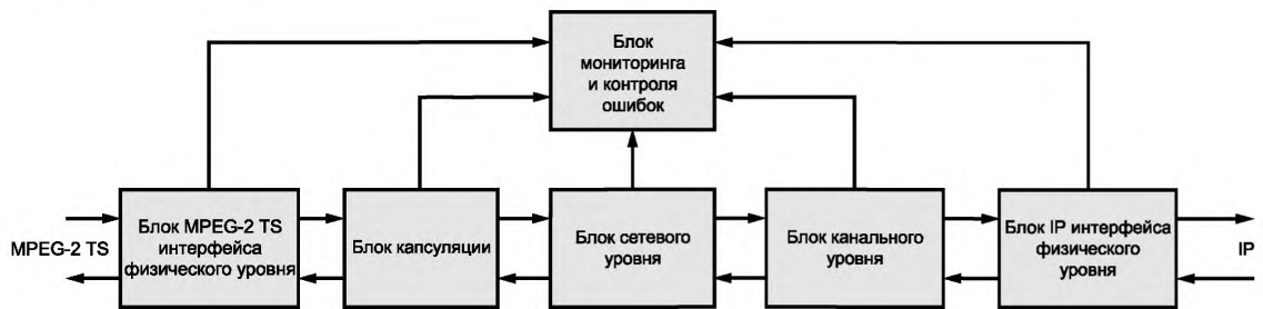
Рисунок 1 — Структурная схема конвертора MPEG-2TS↔IP
