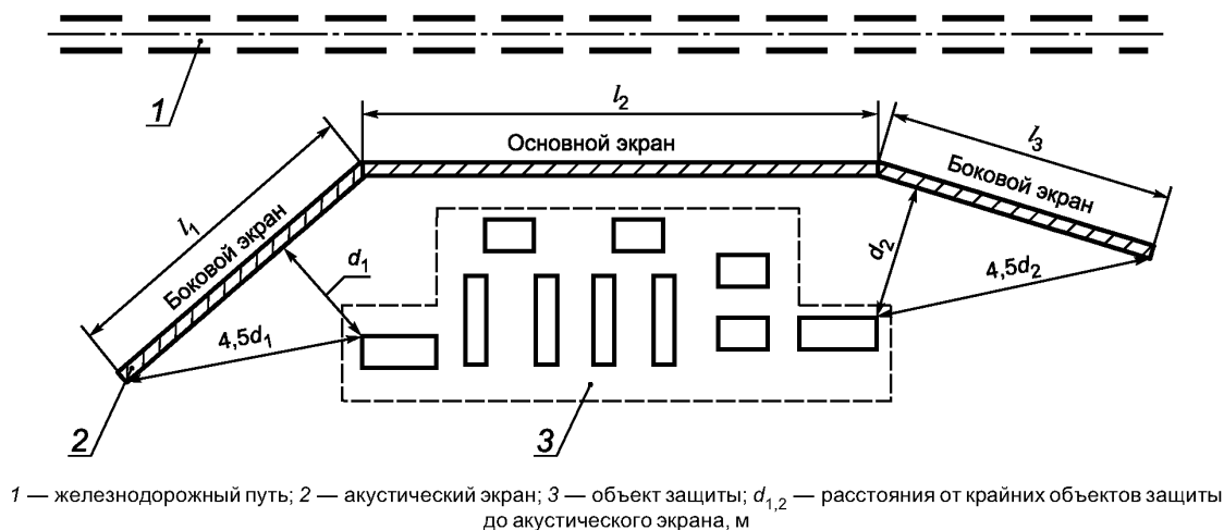
Рисунок 3 — Схема определения длины боковых акустических экранов
