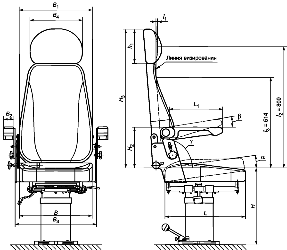
Рисунок 1 — Конструктивные параметры кресла с подголовником
