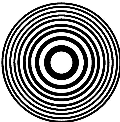
Рисунок 13 — Кольца Ньютона
