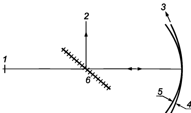
1 — излучатель; 2 — наблюдатель; 3 — воздушный зазор; 4 — испытываемая поверхность V ; 5 — пробная поверхность M (пробное стекло); 6 — светоделитель
