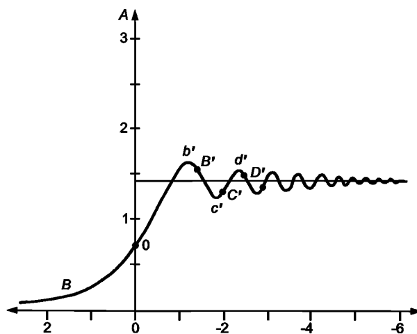
Рисунок 5 — Изменение фазового угла между точками b' и B' при наличии дифракции Френеля на резком крае
