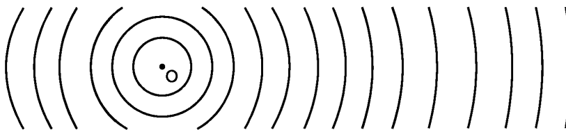
Рисунок 3 — Сферические волны
