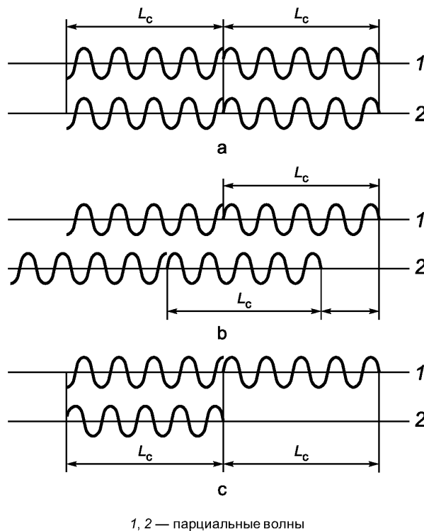
Рисунок 10 — Два следующих друг за другом цуга парциальных волн
