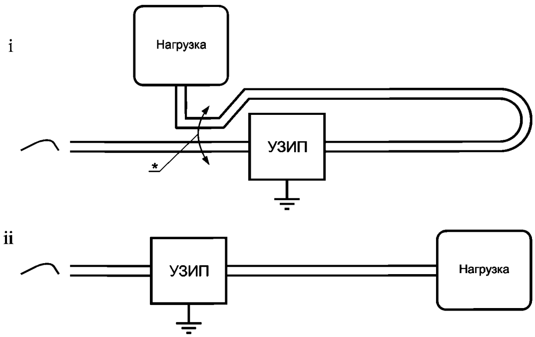
i — неправильная установка — индуктивная связь устанавливается в точке, помеченной звездочкой; ii — правильная установка — кабели до и после УЗИП разделены
