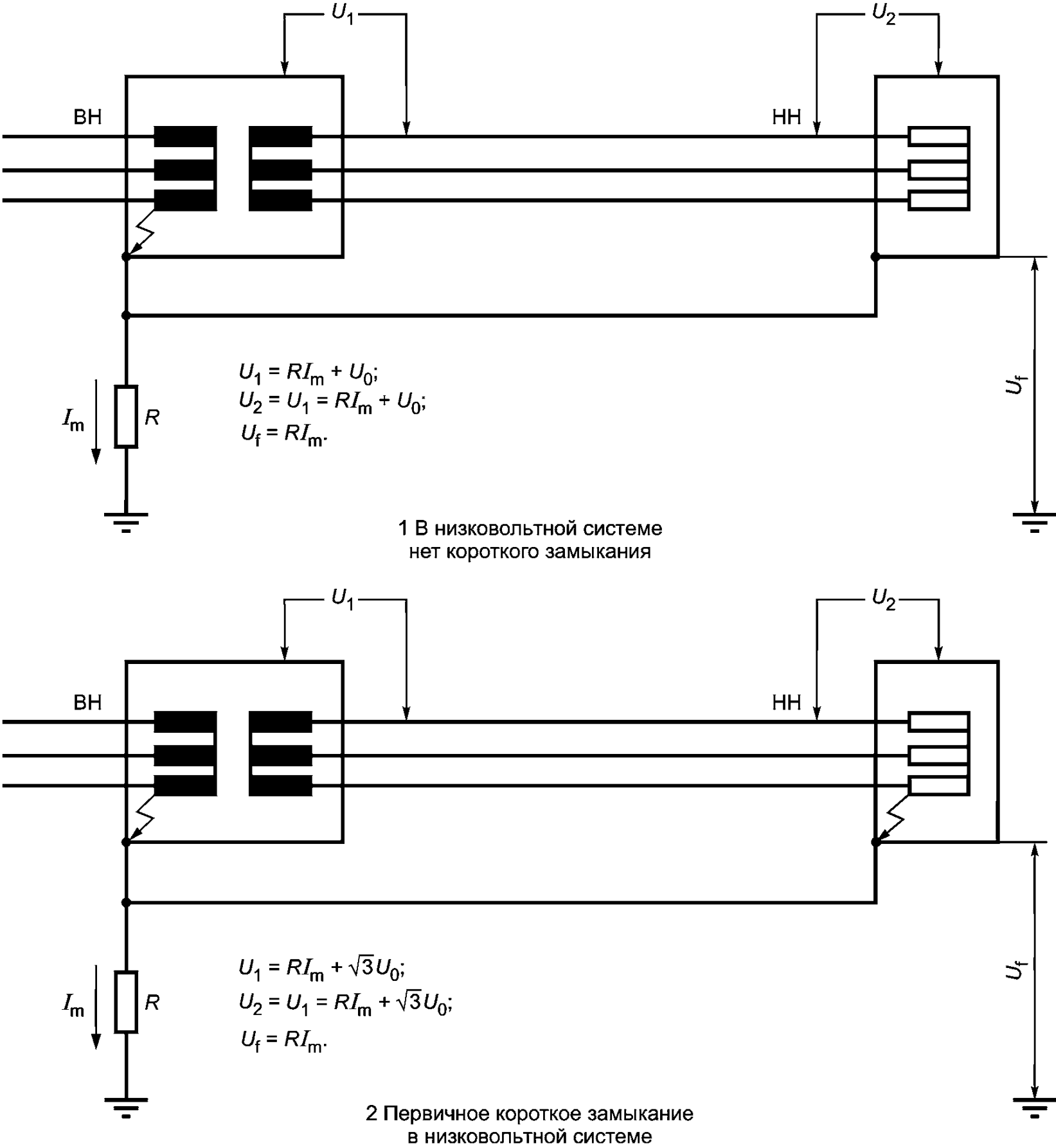
Рисунок Е.10 — Система IT, пример е2
