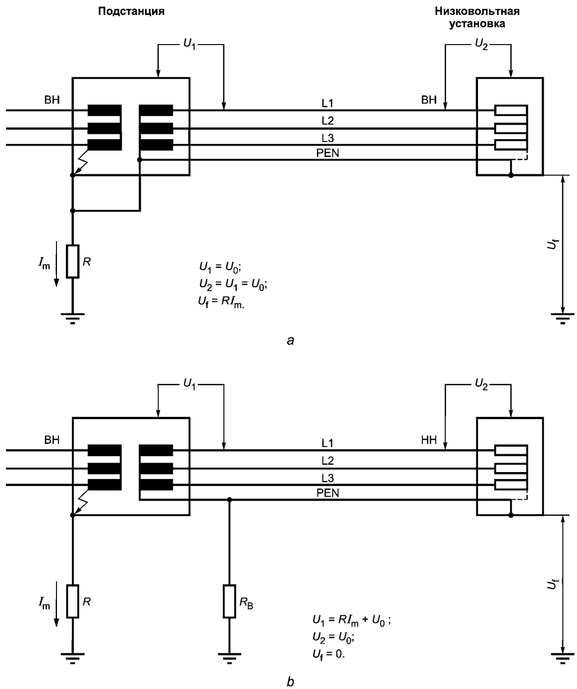
Рисунок Е.2 — Системы TN
