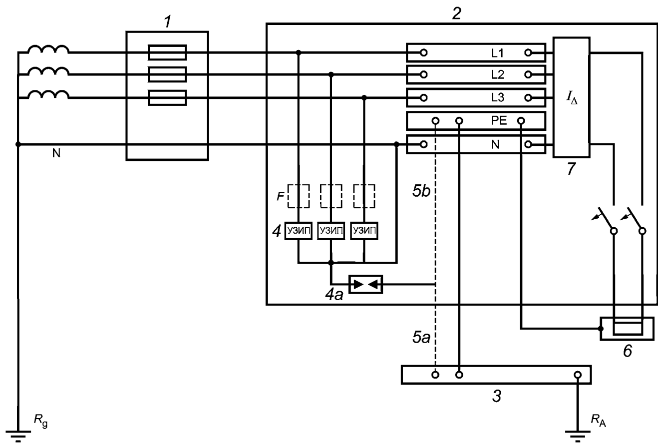
1 — начало электроустановки; 2 — распределительный щит; 3 — главный зажим заземления или шина; 4 — устройства для защиты от импульсных перенапряжений; 4a — устройство для защиты от импульсных перенапряжений согласно МЭК 60364-5-534 или искровой разрядник; 5a, 5b — варианты присоединения УЗИП к заземлению; 6 — оборудование, подлежащее защите; 7 — устройство защиты от дифференциального тока (УДТ); F — защитное устройство, указанное изготовителем УЗИП (например, плавкий предохранитель, автоматический выключатель, УДТ); R_A — заземляющий электрод (заземляющее сопротивление) установки; R_g — заземляющий электрод (заземляющее сопротивление) системы питания
