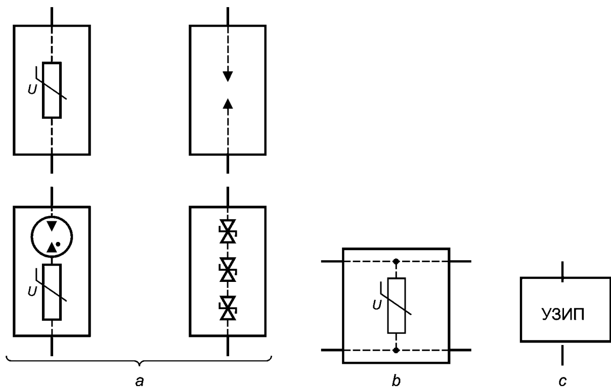
a — однофазные УЗИП; b — однофазное УЗИП с отдельными входными и выходными клеммами; c — общий символ обозначения однофазного УЗИП
