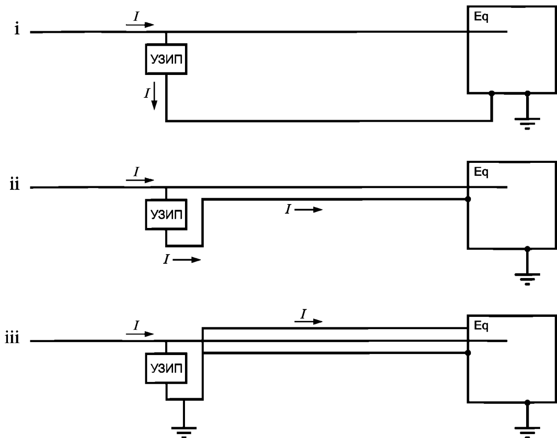
i — плохой вариант из-за большой площади витков — результат высокое d_\phi/d_t вызванное dI/dt ; ii — лучший вариант — малая площадь витков — результат низкое d_\phi/d_t ; iii — самый лучший вариант — экранирование кабеля приводит к d_\phi/d_t = 0 внутри экрана
