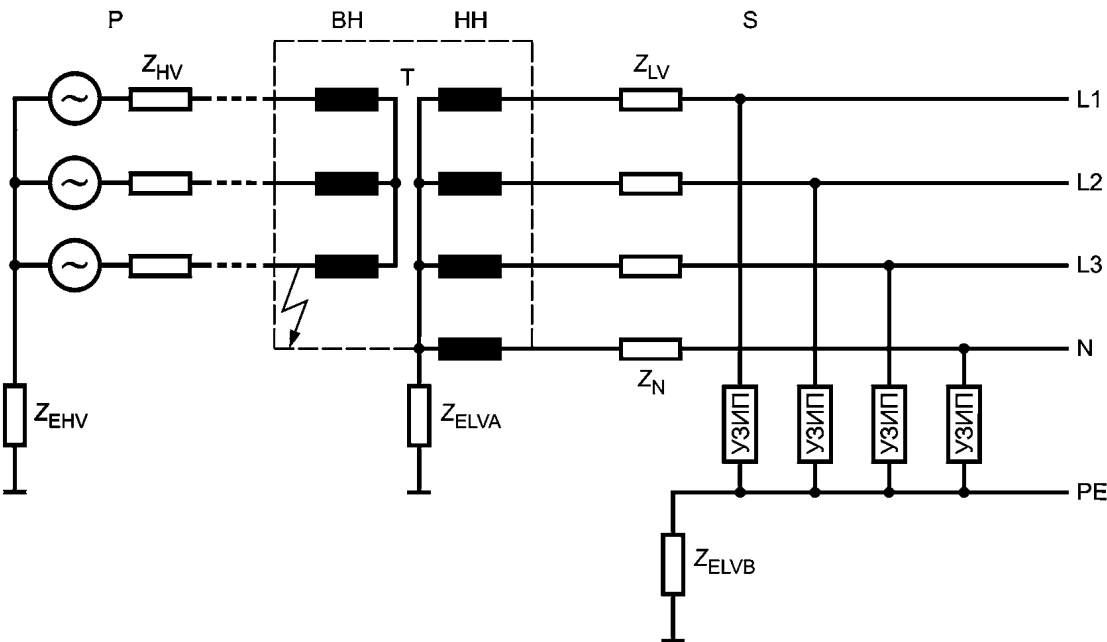
P — BH система высокого напряжения; S — НВ система низкого напряжения; Т — трансформатор
