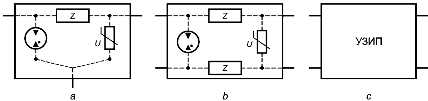
a — двухфазное УЗИП с тремя выводами; b — двухфазное УЗИП с четырьмя выводами; c — общий символ обозначения двухфазного УЗИП; Z — полное сопротивление, включенное последовательно между входными и выходными клеммами
