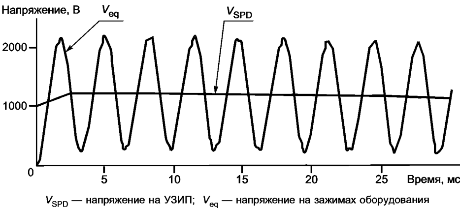
Рисунок К.10 — Пример удвоения напряжения
