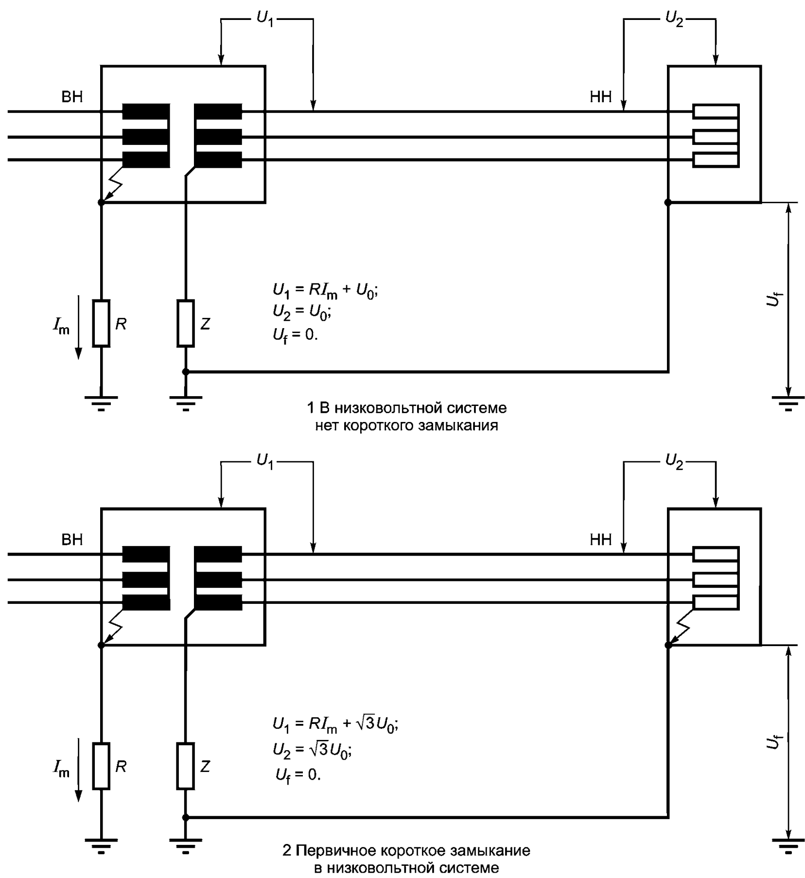
Рисунок Е.8 — Система IT, пример d
