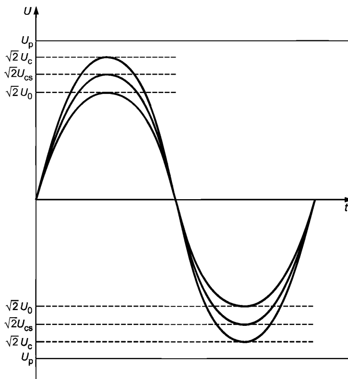
Рисунок 6 — Взаимосвязь между U_p , U_0 , U_c и U_{cs}
