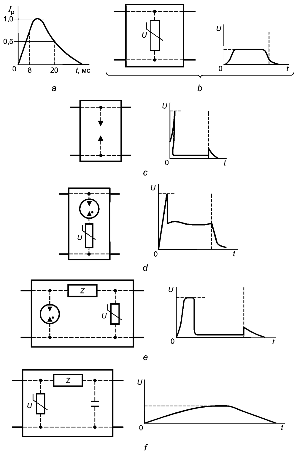
а — форма прикладываемого импульса комбинированной волны; б — форма ограничения прикладываемого импульса УЗИП ограничивающего типа; с — форма ограничения прикладываемого импульса УЗИП коммутирующего типа; д — форма ограничения прикладываемого импульса однопроводным УЗИП комбинированного типа; е — форма ограничения прикладываемого импульса двухпроводным УЗИП комбинированного типа; ф — форма ограничения прикладываемого импульса двухпроводным УЗИП ограничивающего типа с развязывающим фильтром
