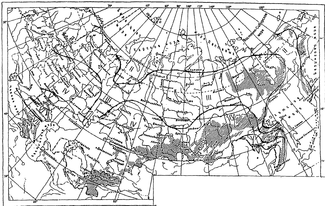
Рисунок А.4 – Схематическая карта районирования по величине удельной энтальпии I , Дж/кг, наружного воздуха в теплый период года (параметры А): I – I = 40 ; II – I = 40 - 43,6 ; III – I = 43,6 - 48,4 ; IV – I = 48,4 - 52,6 ; V – I = 52,6 - 56,8 ; VI – I = 56,8 - 61 ; VII – I = 61 - 65
