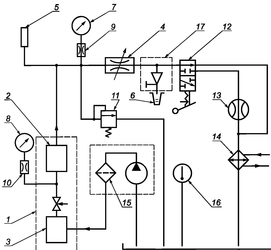
Гидравлическая схема стенда для испытаний насосных станций механизированных крепей
