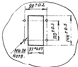
Разметка для монтажа прибора ТЭЛПЗ поз. 5
