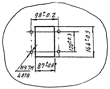
Разметка для монтажа привора ТЭПЗ поз. 5
