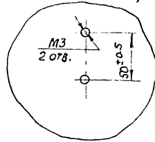
Разметка для крепления реле поз. 16, 17
