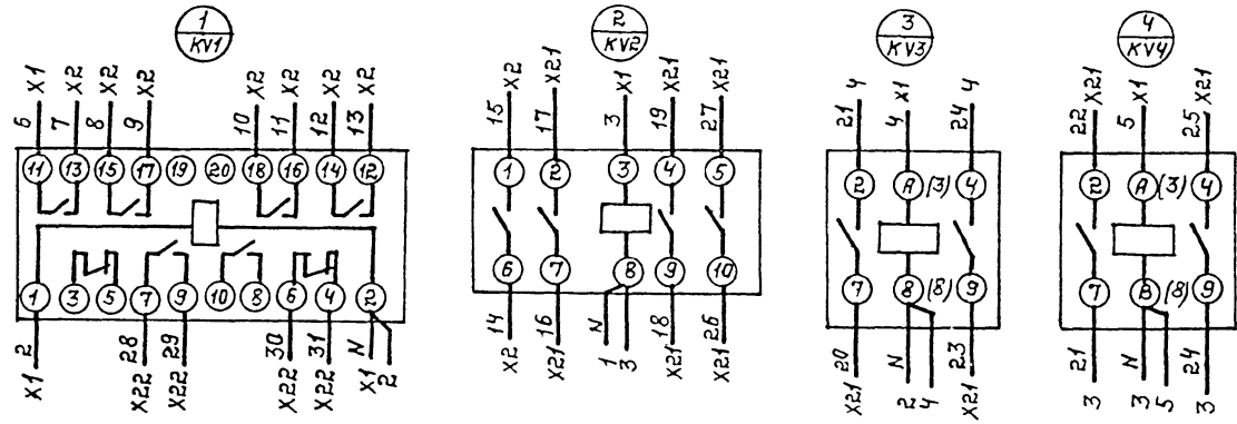
ВИД СПЕРЕДИ.
