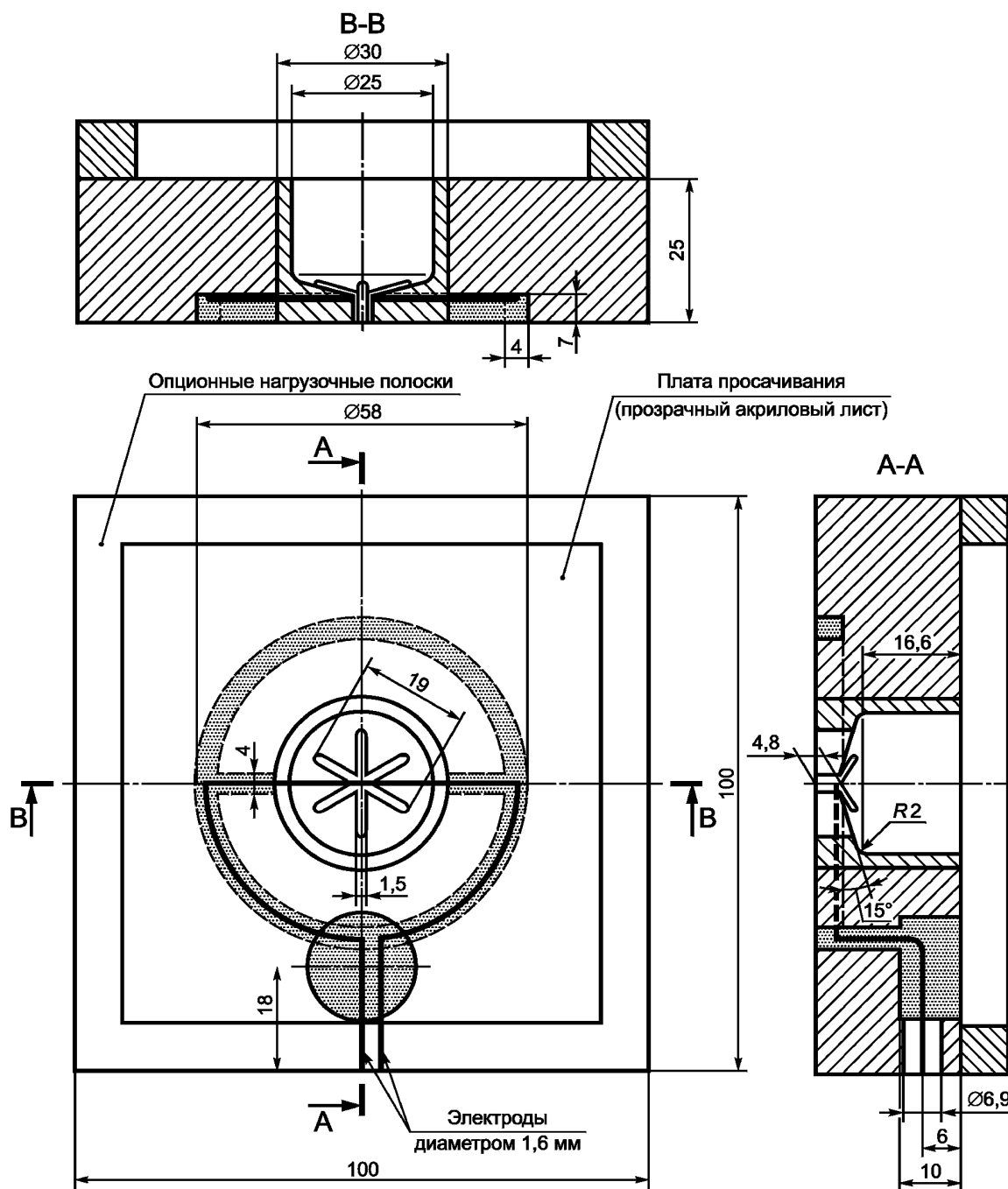
Рисунок 1 — Плата просачивания
