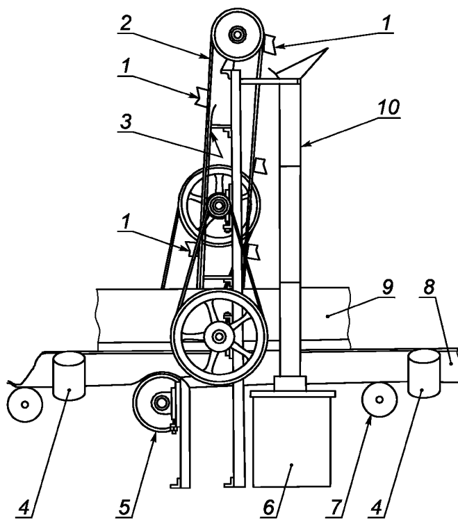
1 — ковш(и) для отбора проб; 2 — лента (цепь) с ковшом для отбора проб; 3 — направляющая цепи ковшей; 4 — баланс; 5 — специальный ролик; 6 — контейнер для проб; 7 — ведущий ролик; 8 — конвейерная лента; 9 — ограждение; 10 — бункер
