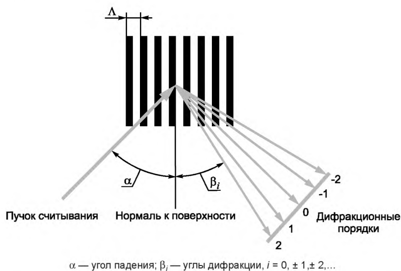
Рисунок А. 2 — Дифракция пучка считывания на дифракционной решетке
