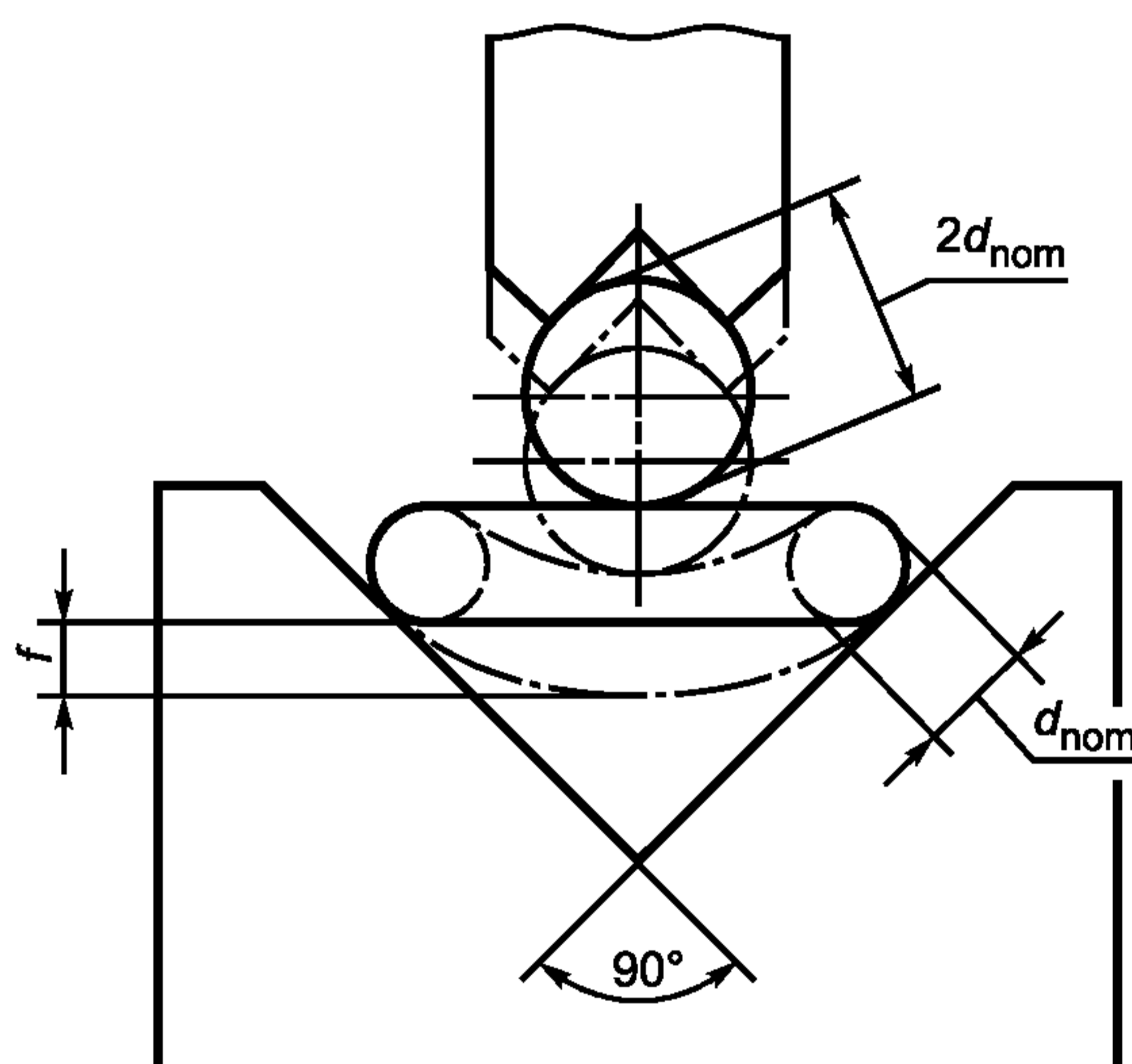
Рисунок 1 — Прогиб f
