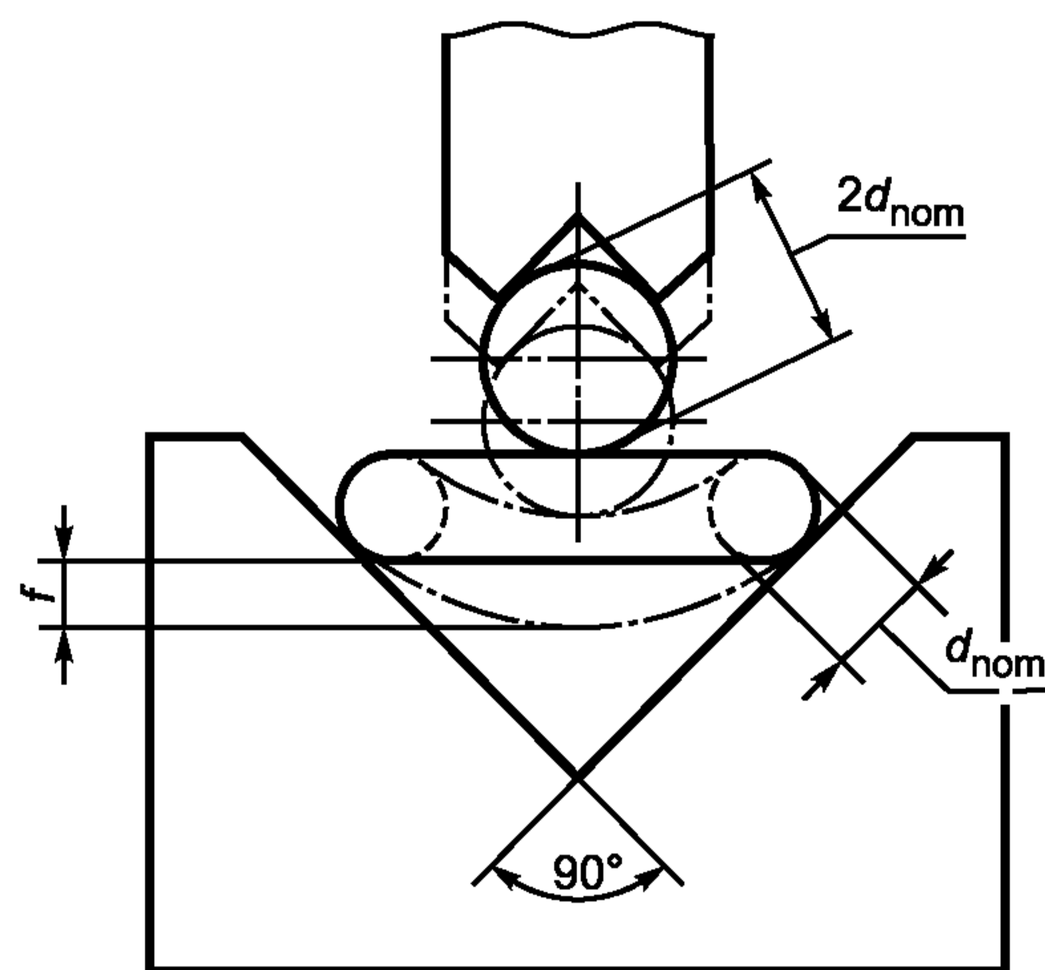
Рисунок 1 — Прогиб f
