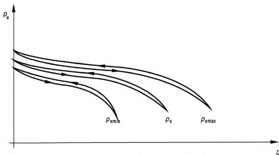
Рисунок 2 — Кривая ( p_{as} — постоянная, p_e — постоянная)
