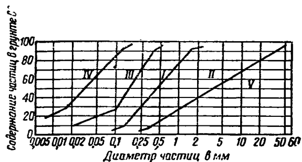
Рис. 2. Группы грунтов, используемых для намыва плотин
