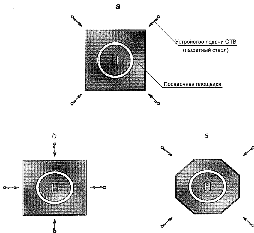
Рисунок А.1 — Схемы размещения стационарных лафетных стволов
