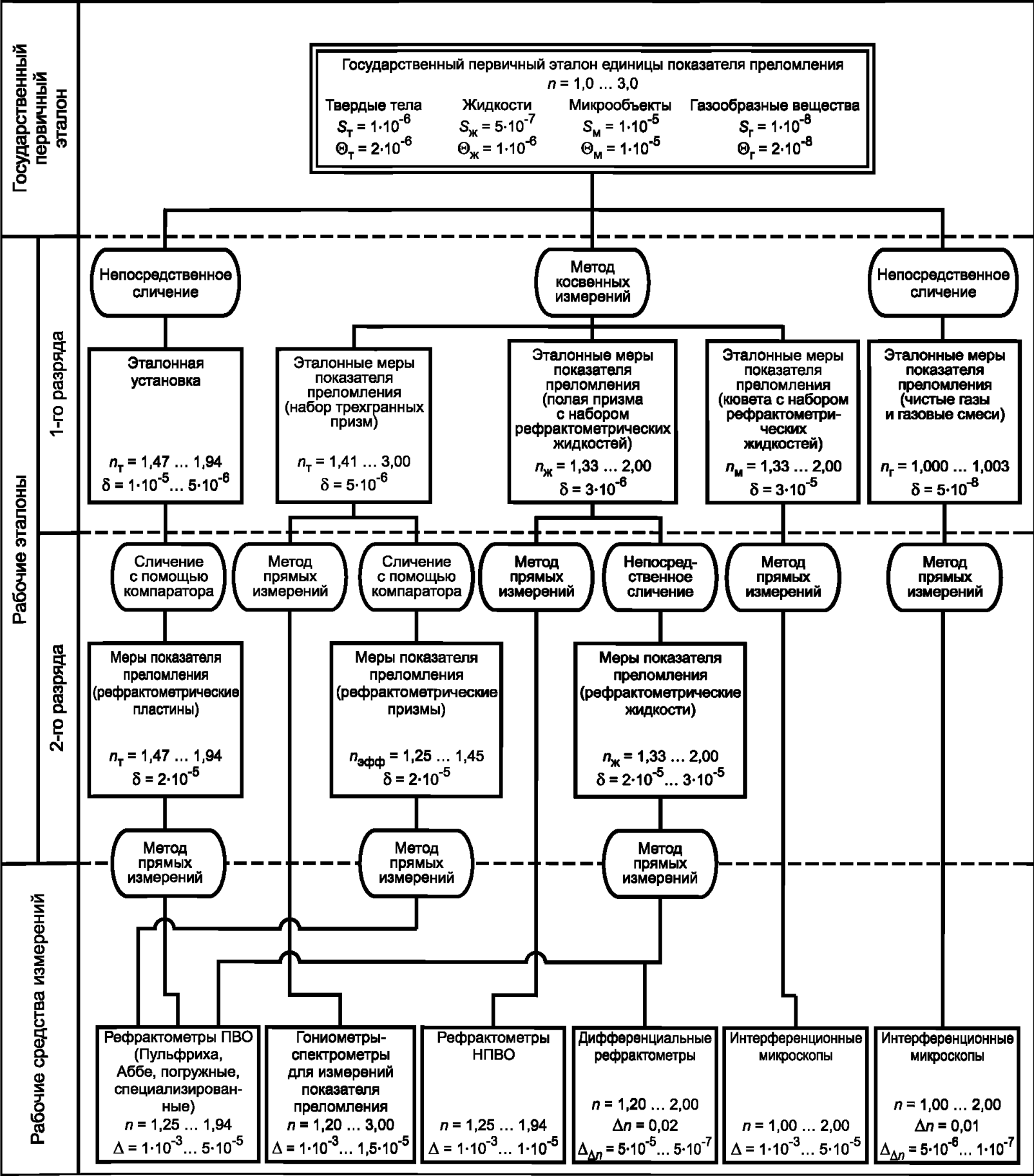
Государственная поверочная схема для средств измерений показателя преломления
