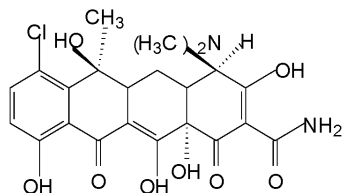
4 - эптитетрациклин
