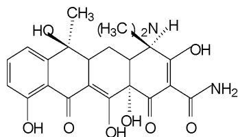
4 - эптитетрациклин
