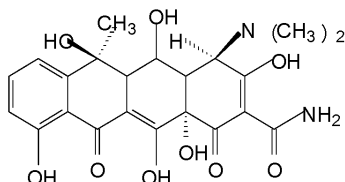
4 - эпикситетрациклин
