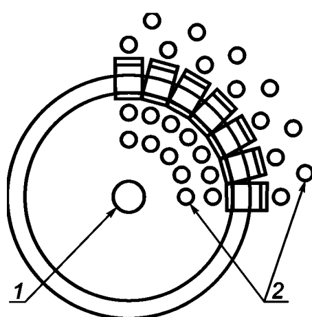
1 — отверстие диаметром 3,3 мм; 2 — vias б) Увеличенная область резисторов
