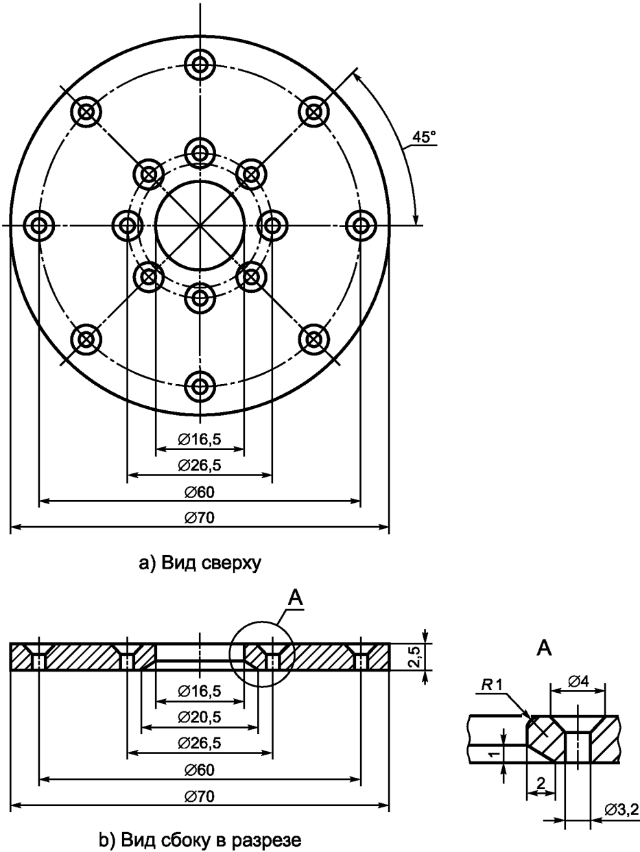
Рисунок В.4 — Коаксиальный датчик. Покрытие: нержавеющая сталь
