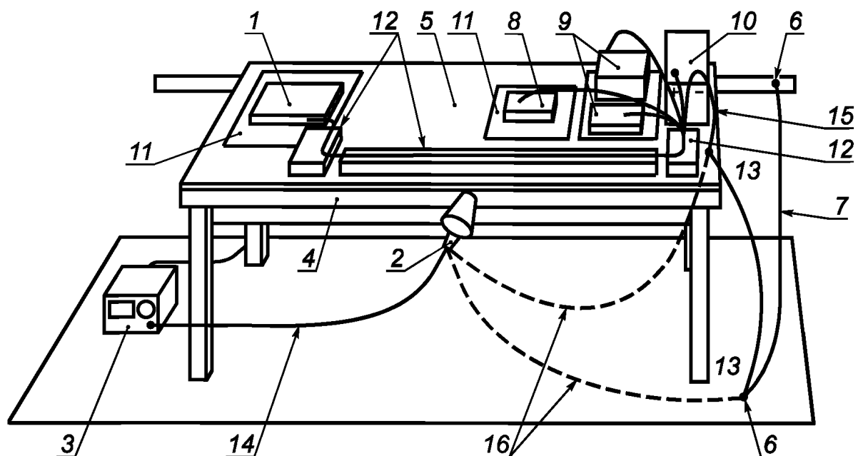
1 — ТС; 2 — испытательный генератор; 3 — основной блок испытательного генератора; 4 — непроводящий стол; 5 — горизонтальная пластина связи; 6 — точка заземления; 7 — соединение с заземлением; 8 — удаленные части ТС; 9 — периферийные устройства; 10 — батарея; 11 — изоляционная пластина (если необходима); 12 — изоляционные подставки; 13 — резисторы 470 кОм; 14 — пластина заземления (дополнительно); 15 — соединение горизонтальной пластины связи с землей; 16 — соединение заземления испытательного генератора с горизонтальной пластиной связи или пластиной заземления (см. программу испытаний)
