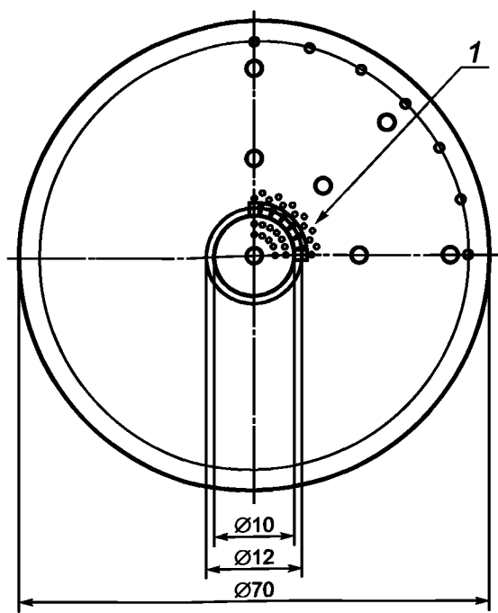
1 — область резисторов, состоящая приблизительно из 25 резисторов (показана только для сектора 90°): а) Печатная плата
