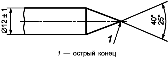
Рисунок 1 — Разрядный наконечник для испытания методом контактного разряда
