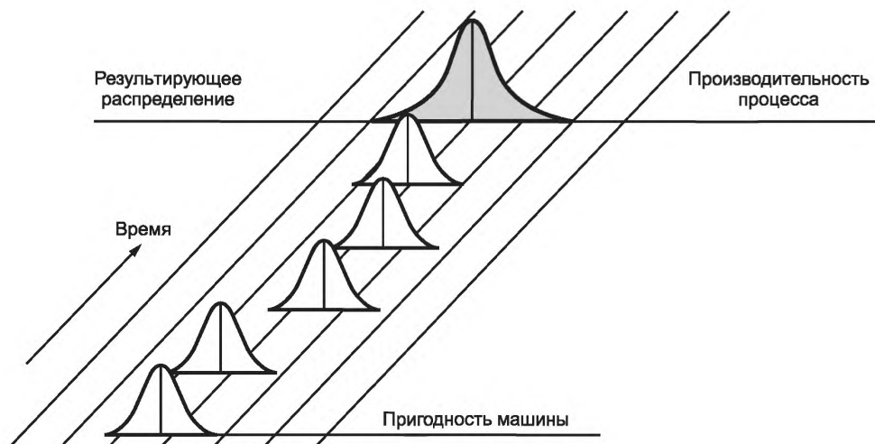
Рисунок 6 — Нестабильный процесс и его пригодность
