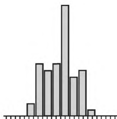
Рисунок 1 — Гистограмма
