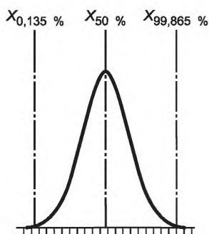
Рисунок 2 — Модель распределения
