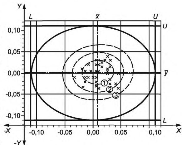
Рисунок 7 — Зона допуска для позиционного допуска
