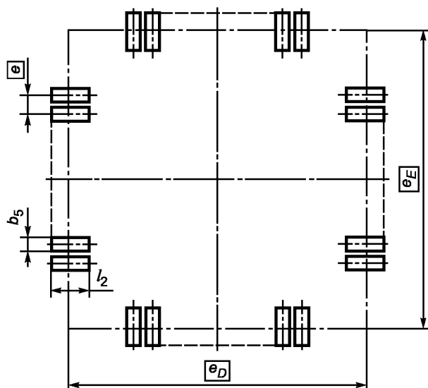
Проекция частей выводов, пригодных для монтажа, на установочную плоскость
