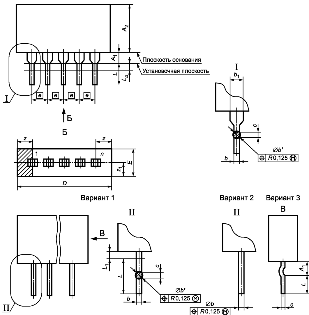
Рисунок 1 — Микросхемы в корпусах подтипа 11
