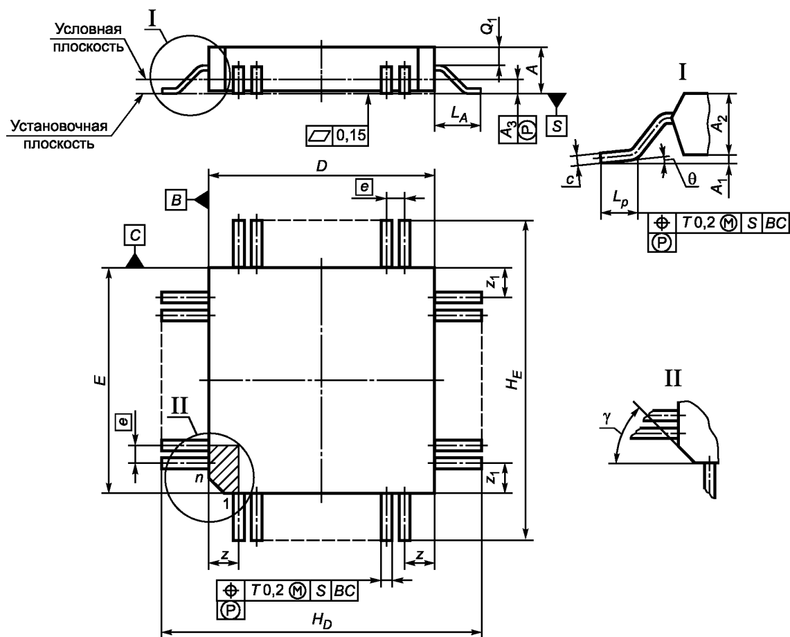
Проекция частей выводов, пригодных для монтажа, на установочную плоскость
