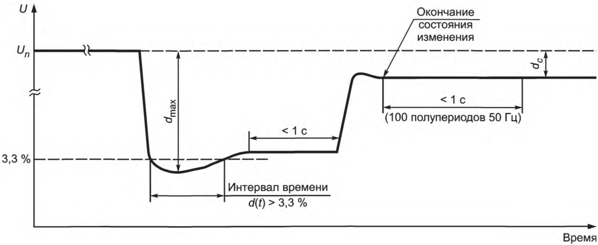
Рисунок В.2а — Пример для объяснения d -параметров
