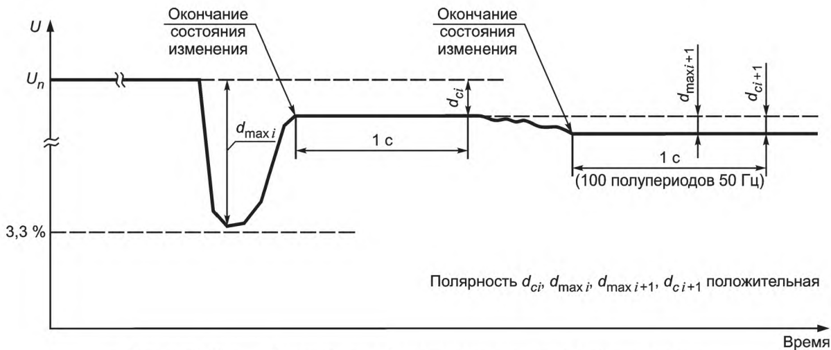
Рисунок В.2b — Пример для объяснения определений d -параметров при многократных установившихся состояниях
