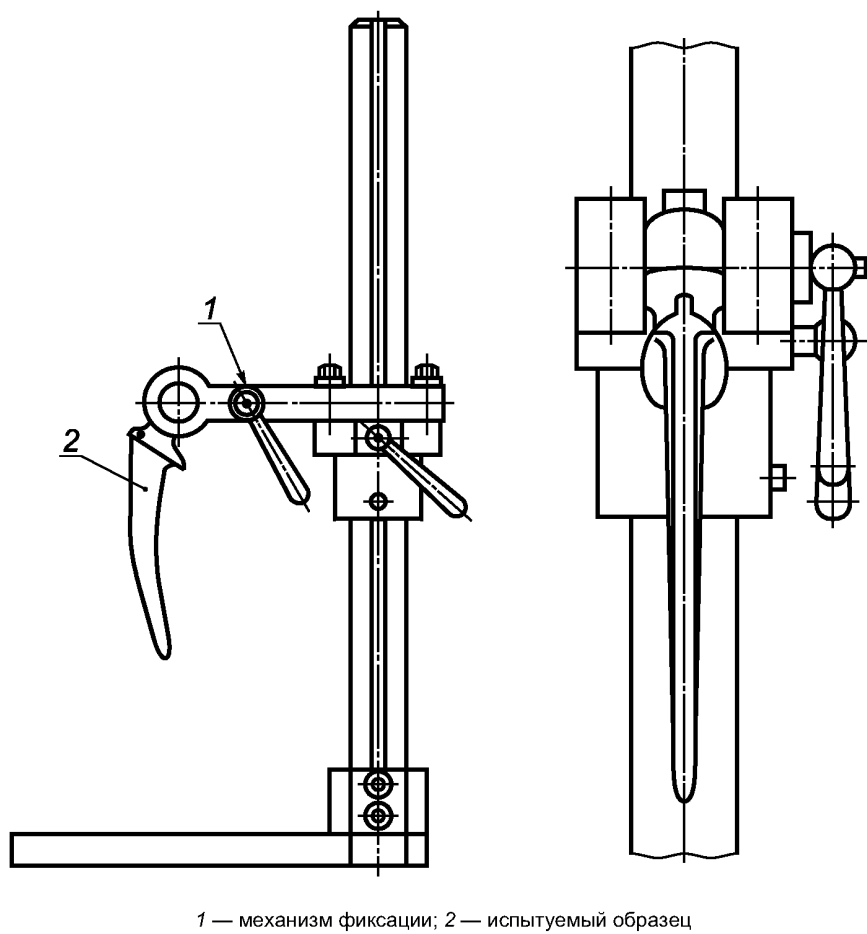
Рисунок А.2 — Пример устройства для захвата головки испытуемого образца при фиксации
